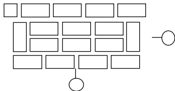
Рис. 60. Кладка простенков толщиной в 2 кирпича
