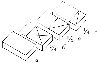
Рис. 2.2. Кирпичи (линиями сверху показаны условные обозначения, принятые в чертежах): a – целый кирпич; б – 3/4 кирпича; в – 1/2 кирпича; г – 1/4 кирпича
