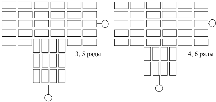
Рис. 56. Кладка примыканий стен толщиной в 2,5 и 2 кирпича
