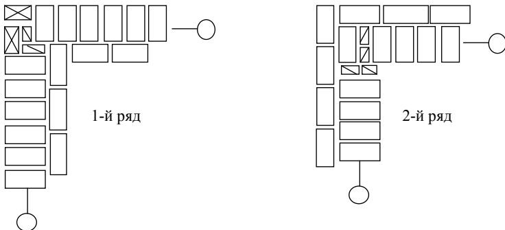
Рис. 2. Кладка углов в 1,5 кирпича
