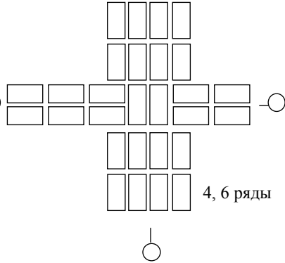
Рис. 42. Кладка пересечений стен толщиной в 2 и 1 кирпич
