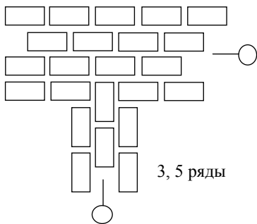
Рис. 54. Кладка примыканий стен толщиной в 2 и 1,5 кирпича
