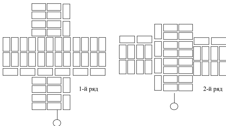
Рис. 8. Кладка пересечений стен толщиной в 2,5 кирпича
