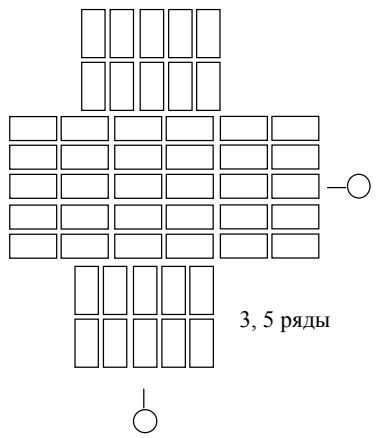
Рис. 40. Кладка пересечений стен толщиной в 2,5 кирпича
