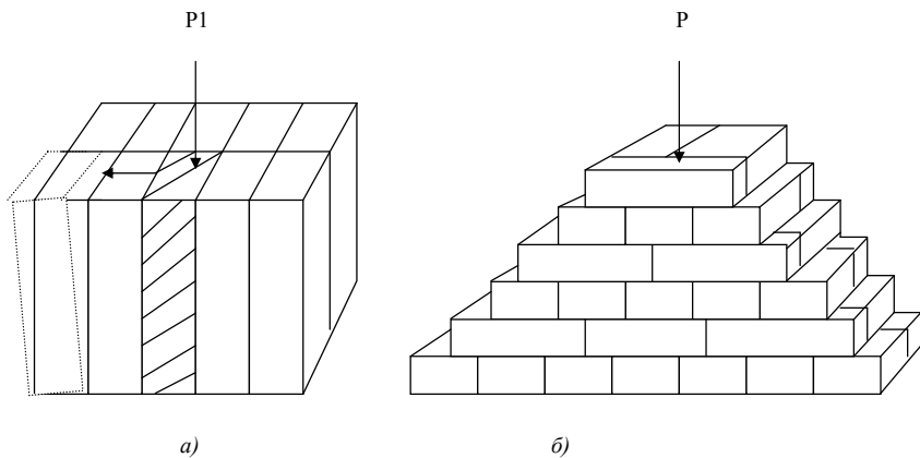
Рис. 1.5. Системы перевязки кладки: a – кладка без перевязки швов; б – кладка с перевязкой швов
