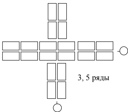
Рис. 37. Кладка пересечений стен толщиной в 1 кирпич
