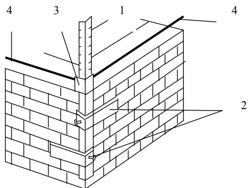
Рис. 1.2. Схема крепления угловой металлической порядовки: 1 – порядовка; 2 – скобы для крепления порядовки; 3 – ползунок для крепления причалки; 4 – шнур-причалка
