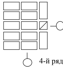
Рис. 68. Кладка столбов сечением 2,5x2,5 кирпича
