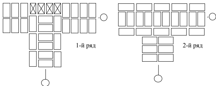
Рис. 17. Кладка примыканий стен толщиной в 2 кирпича
