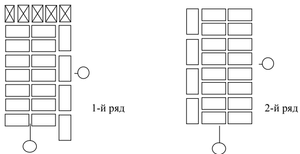
Рис. 28. Кладка вертикальных ограничений толщиной в 2,5 кирпича
