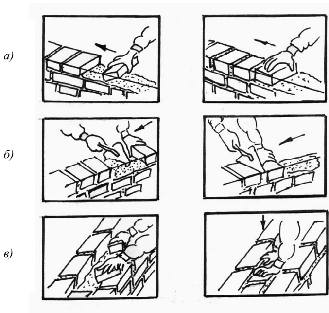
Рис. 2.1. Укладка кирпича: а – впрысык; б – вприжим; в – вполупрысык
