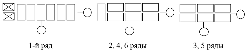
Рис. 62. Кладка вертикальных ограничений толщиной в 1 кирпич
