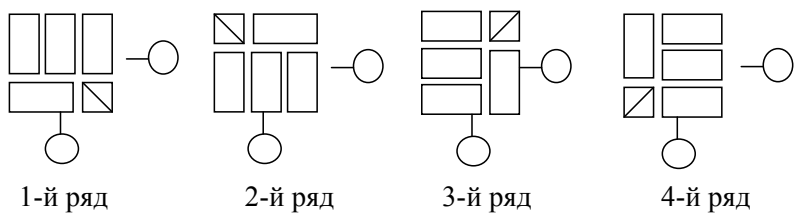
Рис. 66. Кладка столбов сечением 1,5x1,5 кирпича
