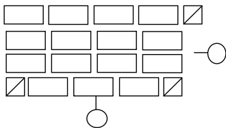
Рис. 60. Кладка простенков толщиной в 2 кирпича
