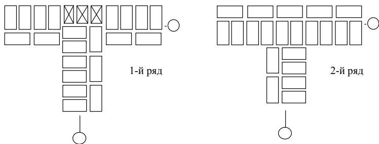
Рис. 16. Кладка примыканий стен толщиной в 1,5 кирпича
