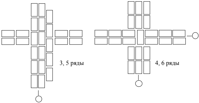
Рис. 41. Кладка пересечений стен толщиной в 1,5 и 1 кирпич
