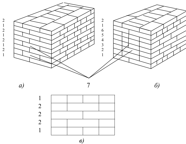
Рис. 1.6. Системы перевязки при кладке стен: a – однорядная (цепная) перевязка; б – многорядная перевязка; в – трехрядная кладка; 1 – тычковый ряд; 2–6 – ложковые ряды; 7 – забутка
