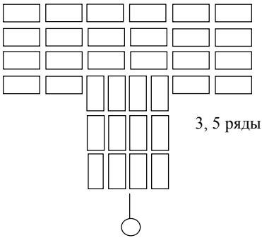
Рис. 49. Кладка примыканий стен толщиной в 2 кирпича
