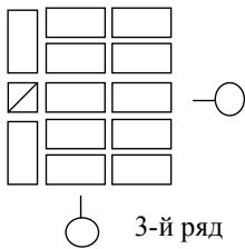
Рис. 68. Кладка столбов сечением 2,5x2,5 кирпича
