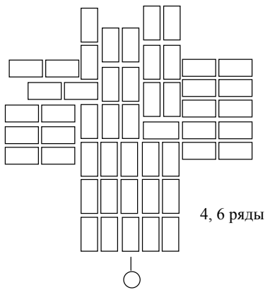
Рис. 40. Кладка пересечений стен толщиной в 2,5 кирпича
