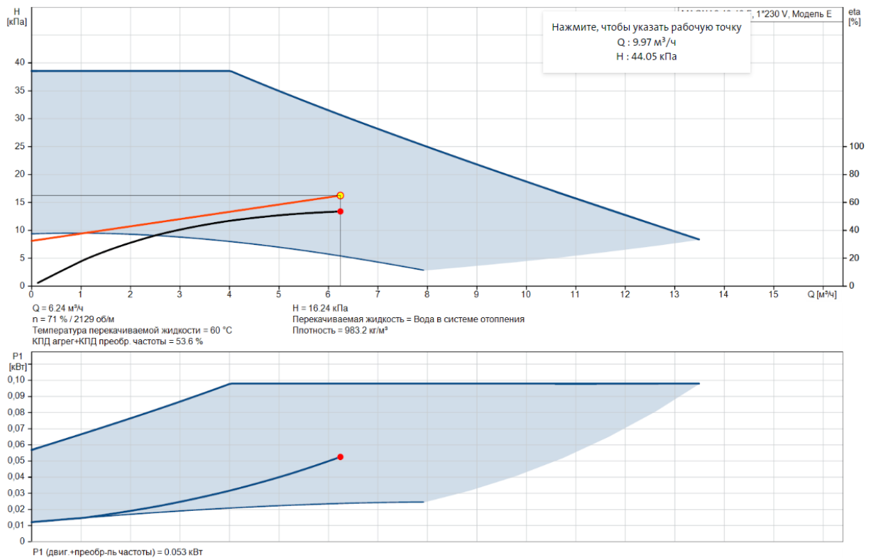
Рисунок 8 – Характеристики насоса GRUNDFOSS MAGNA3 40-40 F
