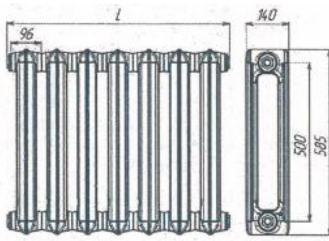
Рисунок 5 – Радиатора МС-140 М4-500
