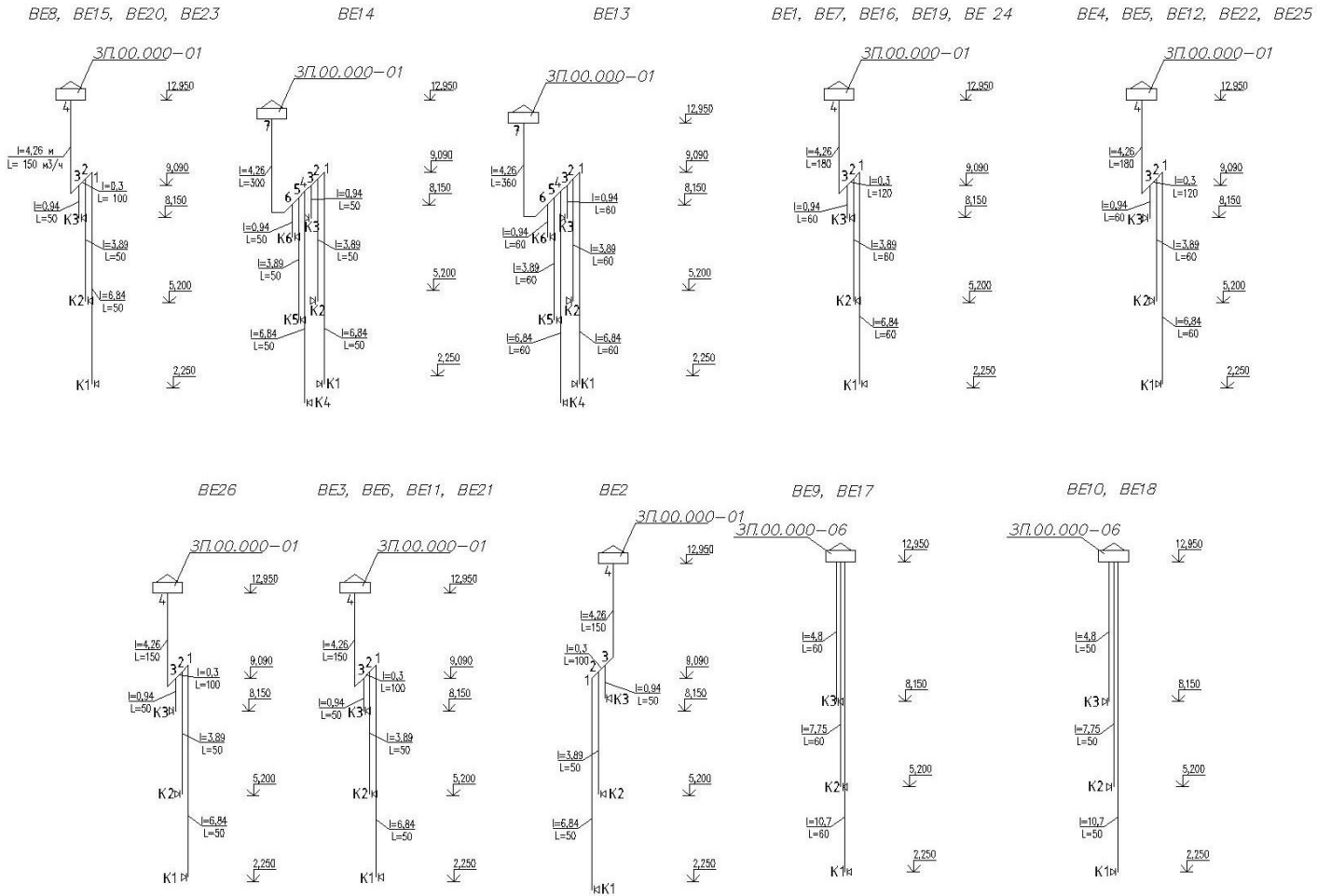
Рисунок В.1 – Расчетные схемы системы естественной вентиляции
