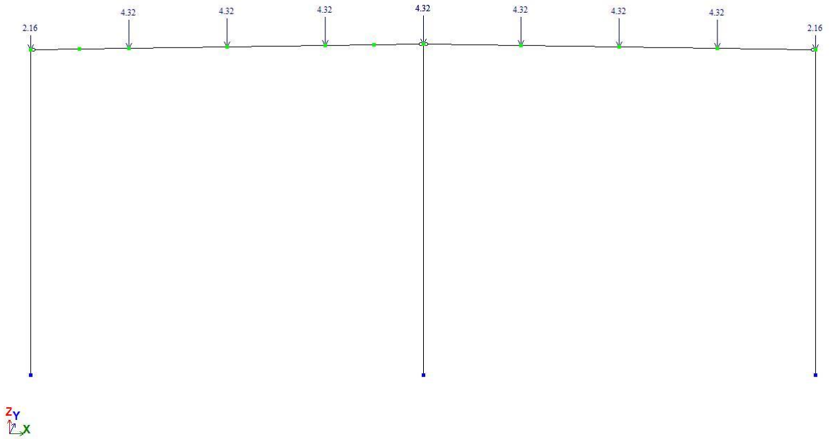
Снеговая нагрузка №2
