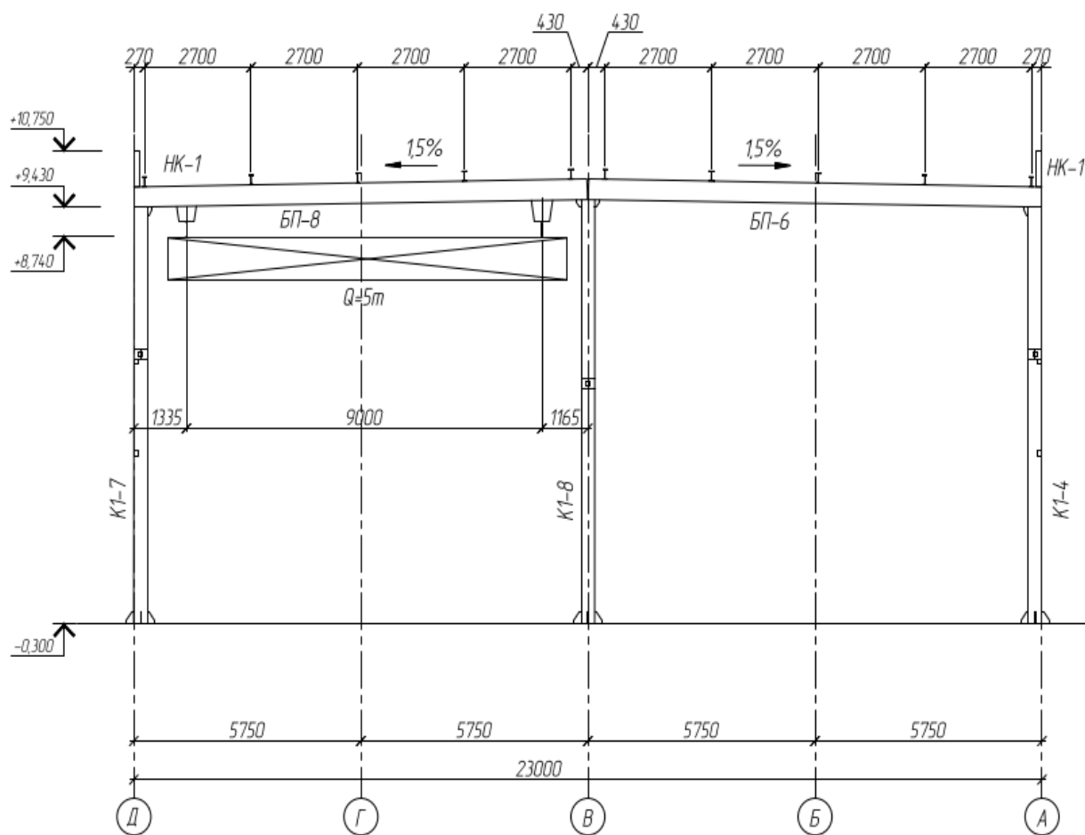
Рисунок 3 – Геометрические размеры рамы
