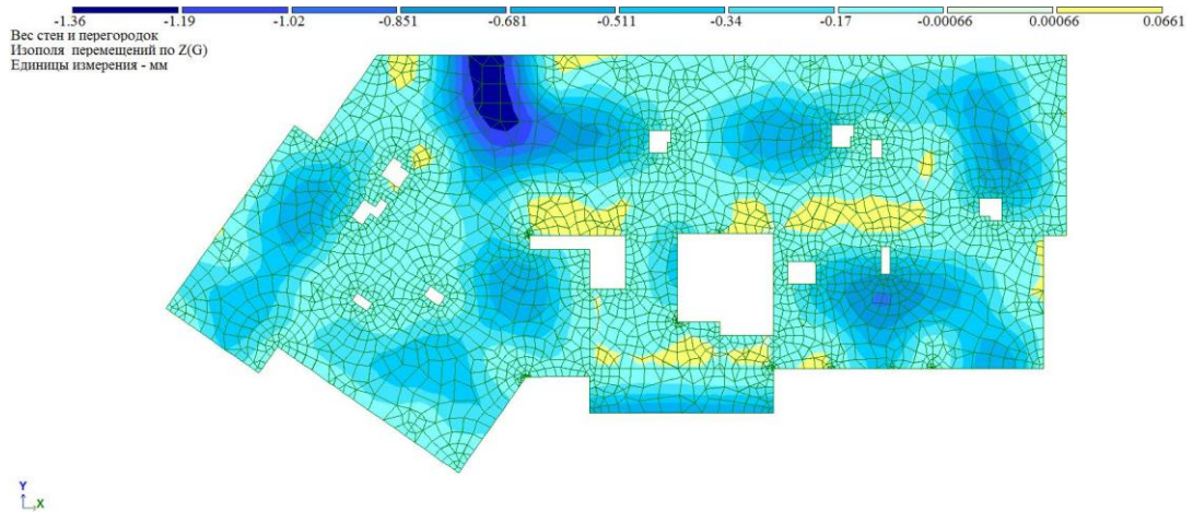
Рисунок Б.11 – «Изополюса перемещения от собственного веса по оси Z = - 10,2 мм» [28].
