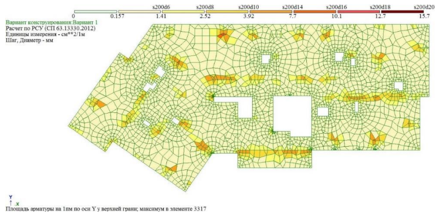
Рисунок Б.10 – «Верхняя арматура в плите перекрытия вдоль оси Y» [28].
