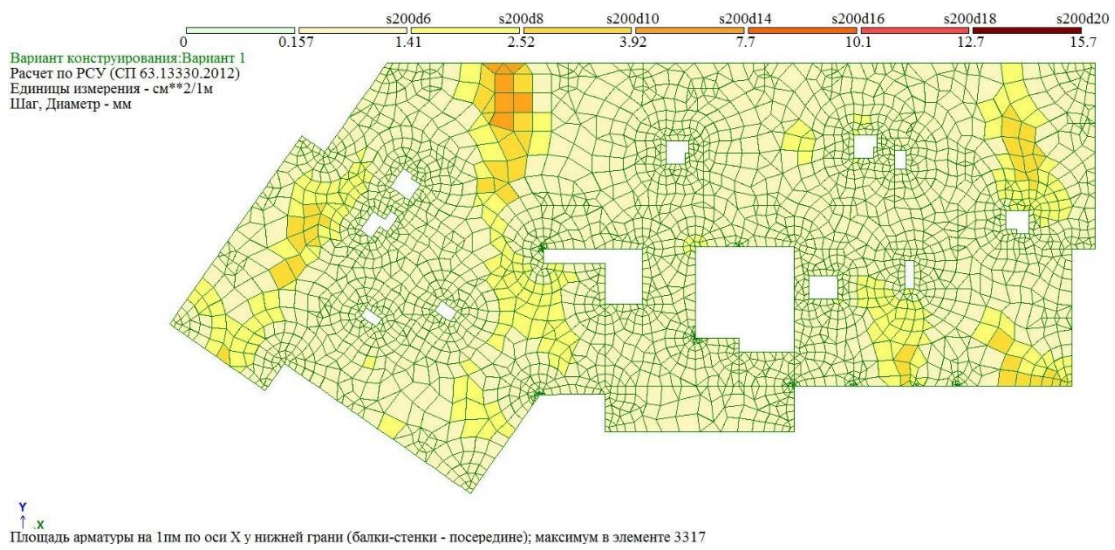
Рисунок Б.7 – «Нижняя арматура в плите перекрытия вдоль оси X» [28].
