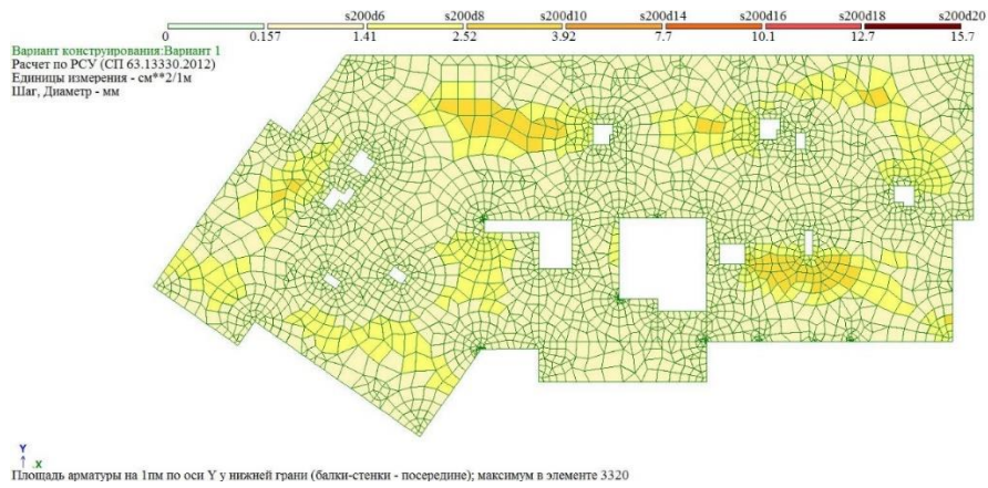
Рисунок Б.9 – «Нижняя арматура в плите перекрытия вдоль оси Y» [28].
