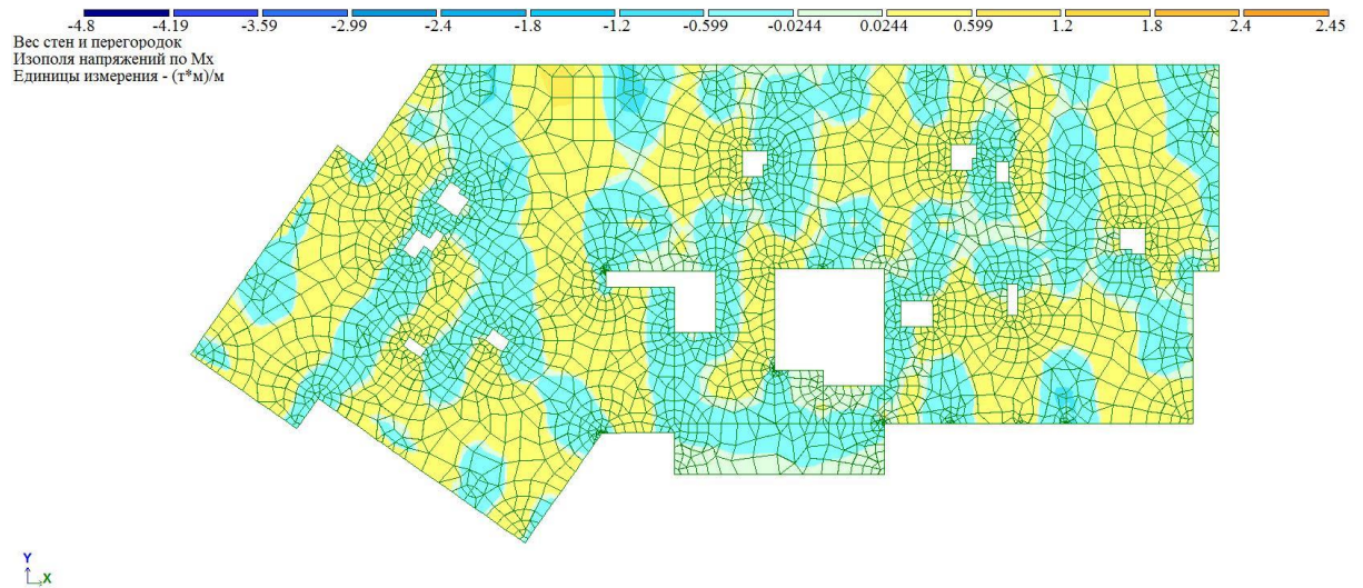
Рисунок Б.5 – «Изополя моментов от собственного веса M_x » [28].
