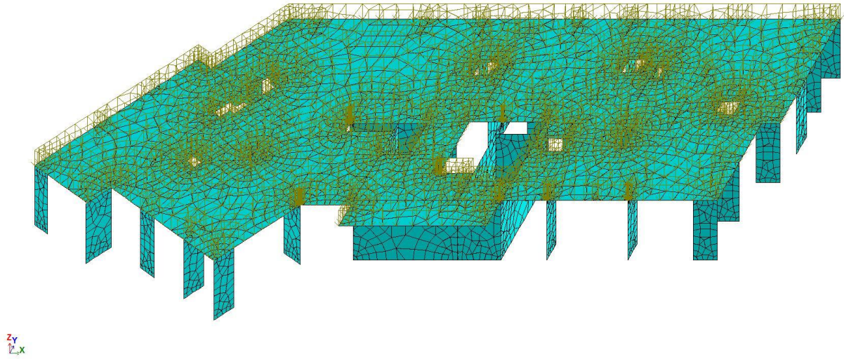
Рисунок Б.3 – Вес полов
