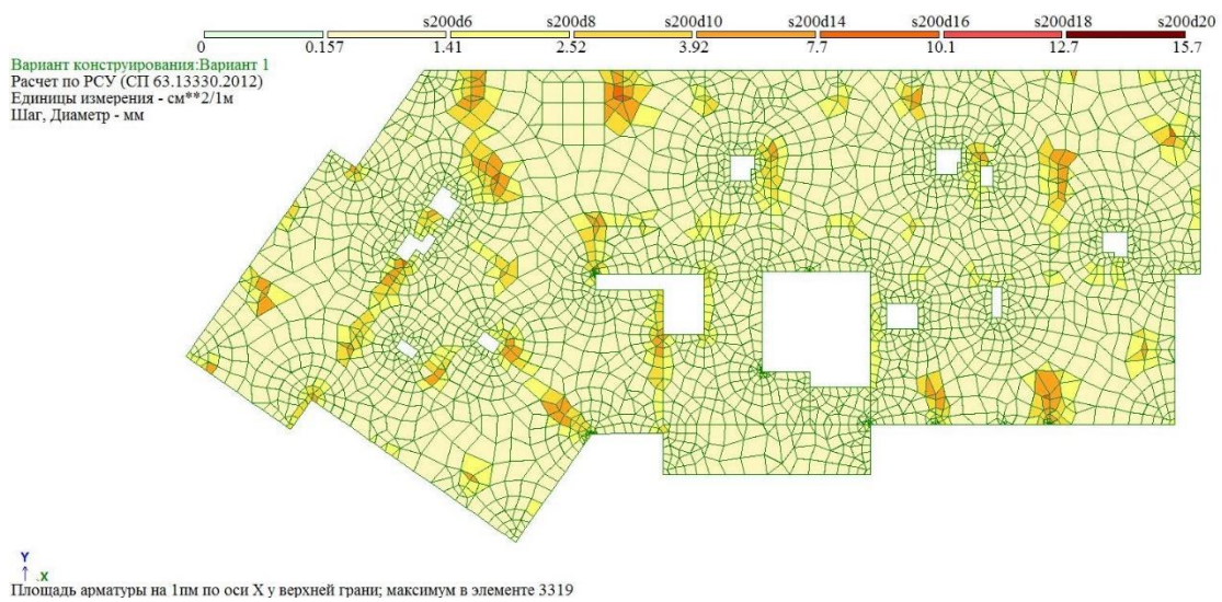
Рисунок Б.8 – «Верхняя арматура в плите перекрытия вдоль оси X» [28].
