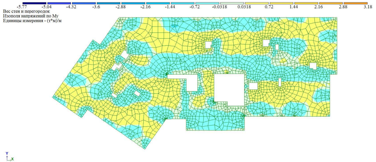
Рисунок Б.6 – «Изополя моментов от собственного веса M_y » [28].
