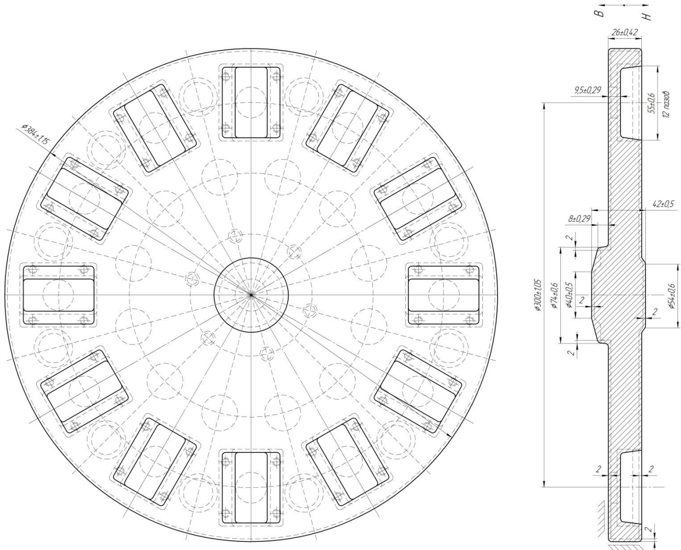
Рисунок 2 – Общий вид отливки
