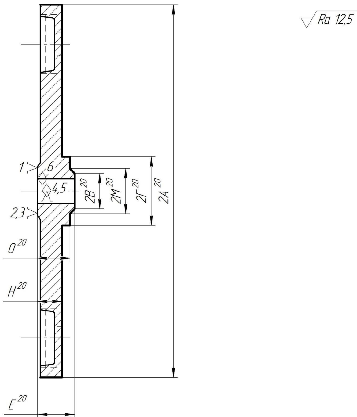
Рисунок 3 – Операционный эскиз операции 020
