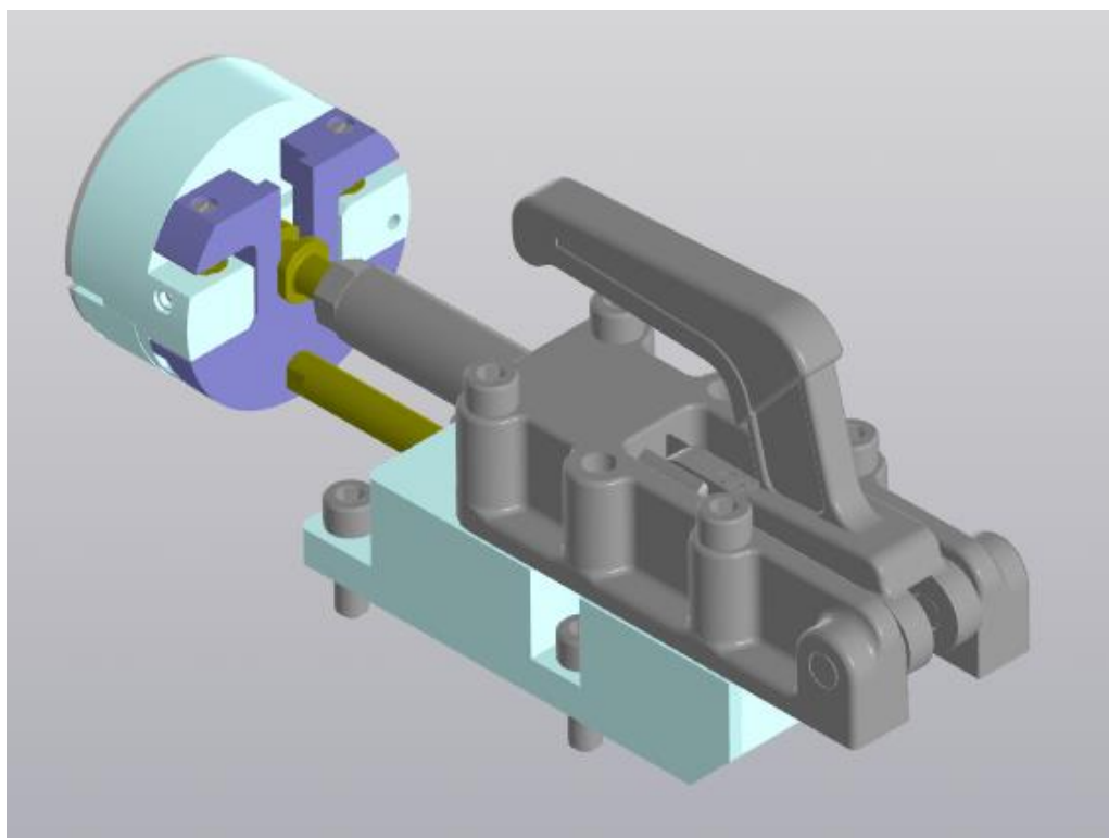
Рисунок 10 – Модернизированная оснастка Н4М для производства катализаторов
