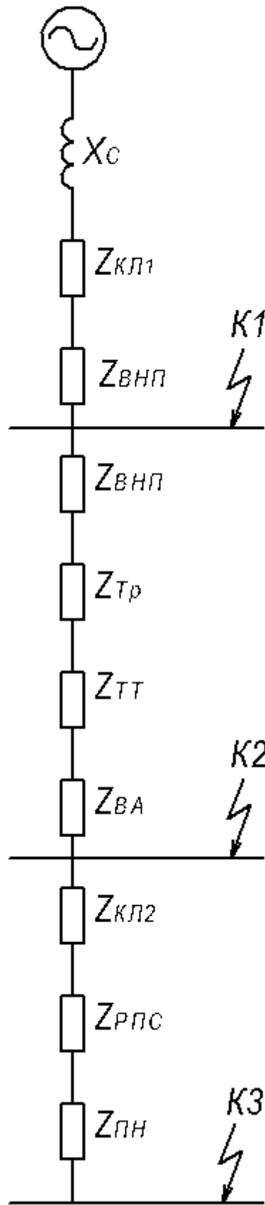
Рисунок 8 – Схема замещения сети
