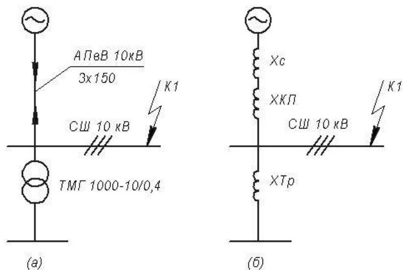
Рисунок 6 - Расчётная схема сети и схема замещения
