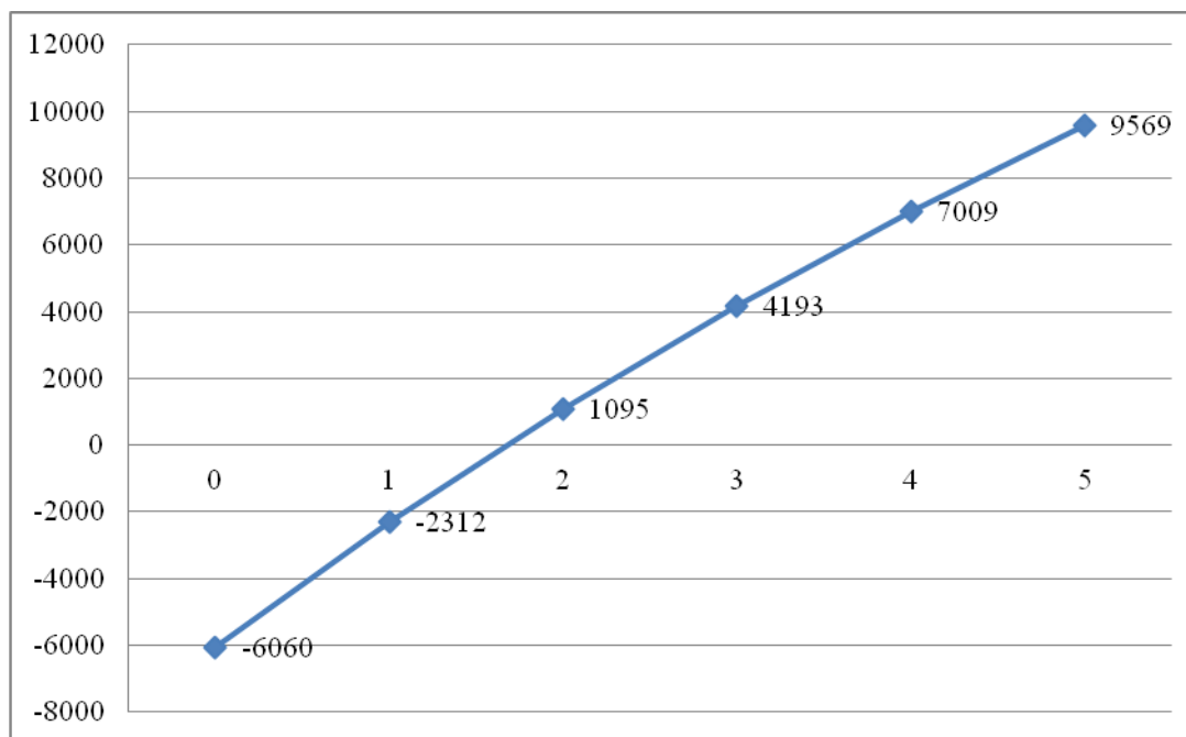
Рисунок 22 – График NPV
