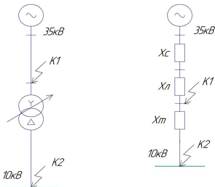
Рисунок 5.1 – Расчетная схема ГПП и ее схема замещения с указанием точек КЗ
