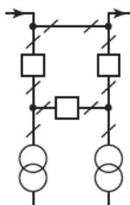
Рисунок 4.1 - Мостик с выключателями в цепях линий и ремонтной перемычкой со стороны линий
