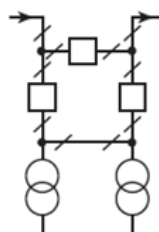
Рисунок 4.2 - Мостик с выключателями в цепях трансформаторов и ремонтной перемычкой со стороны трансформаторов
