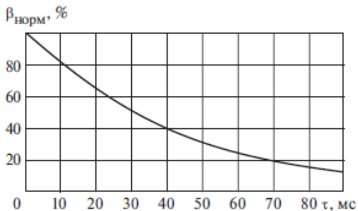
Рисунок 6.1 - Нормированное содержание апериодической составляющей
