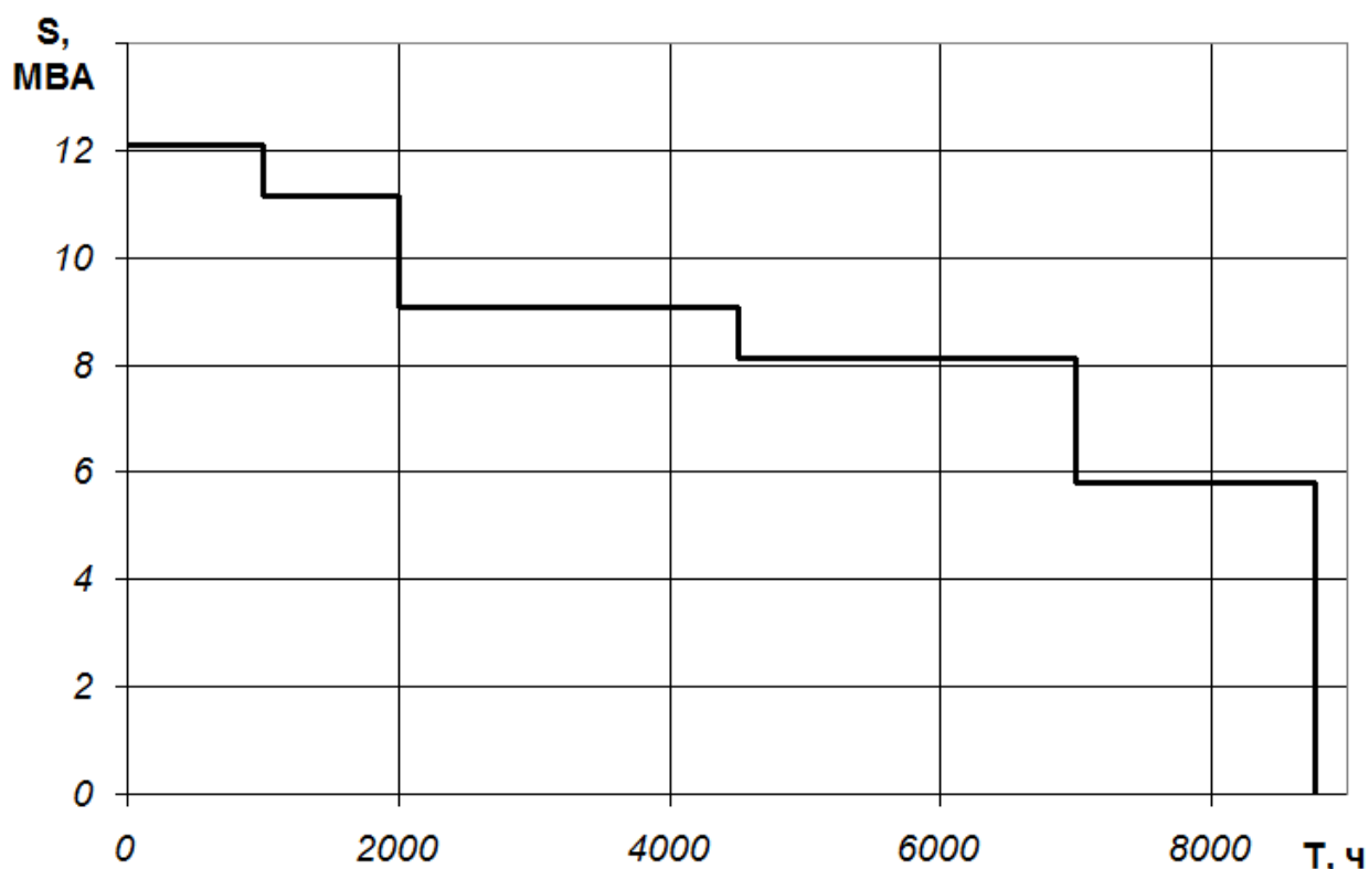
Рисунок 2.1 – Годовой график нагрузки подстанции на трехлетнюю перспективу
