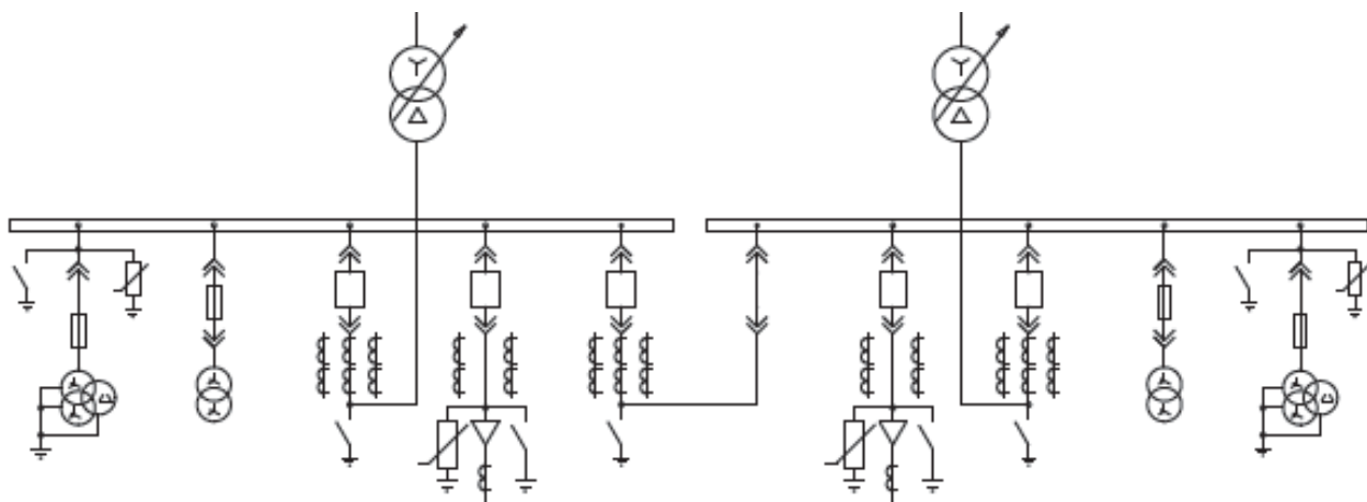
Рисунок 8.1 - Питание ТСН подстанции на постоянном оперативном токе
