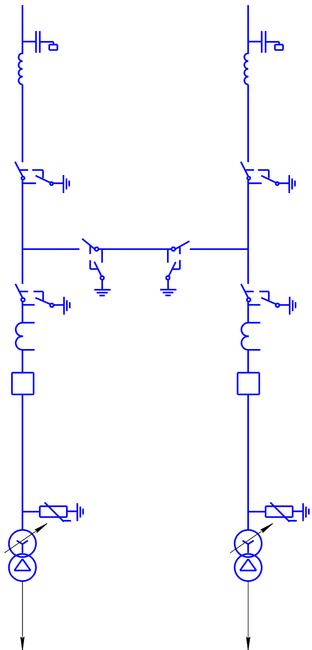
Рисунок 2 – Схема электрическая принципиальная РУ №35-4Н
