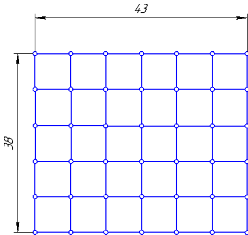
Рисунок 7 – Схема заземляющего устройства
