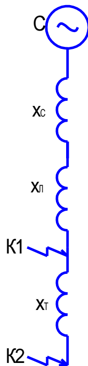
Рисунок 4 – Эквивалентная схема замещения
