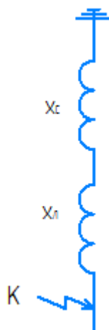
Рисунок 6 – Схема замещения нулевой последовательности
