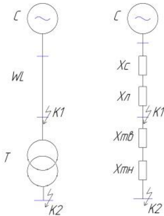
Рисунок 6.1 - Схемы для определения значений токов КЗ – расчетная и схема замещения
