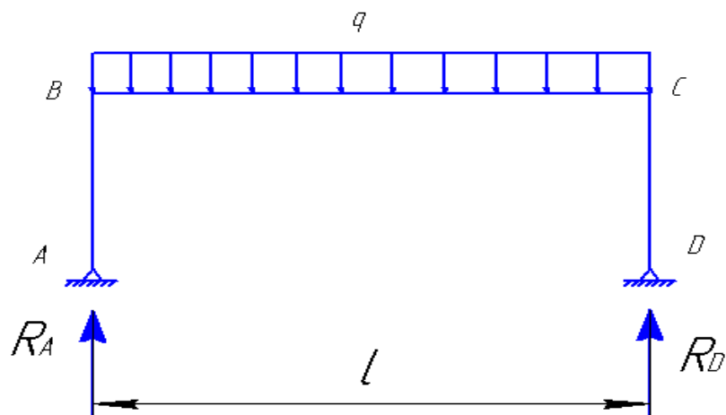
Рисунок 2.8 - Реакция и нагрузка на платформу
