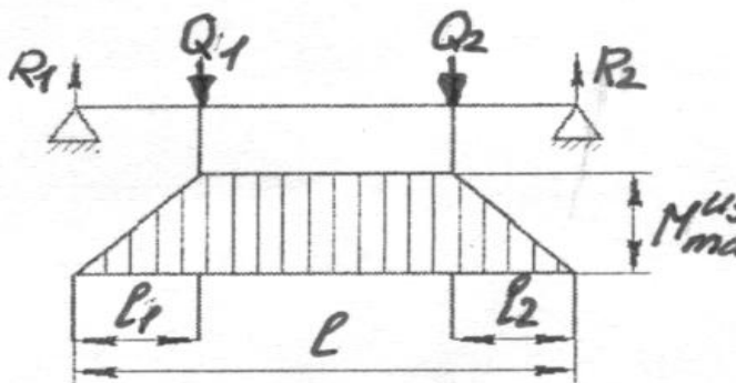
Рисунок 2.10 - Распределенная нагрузка на платформу траверсы
