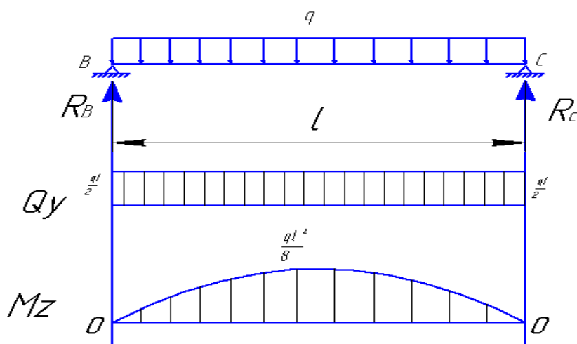
Рисунок 2.9 - Эпюры для расчета на прочность платформы
