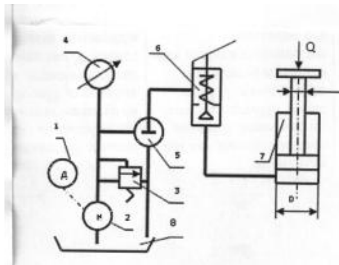
Рисунок 3.3 – Принципиальная гидравлическая схема привода подъемника
