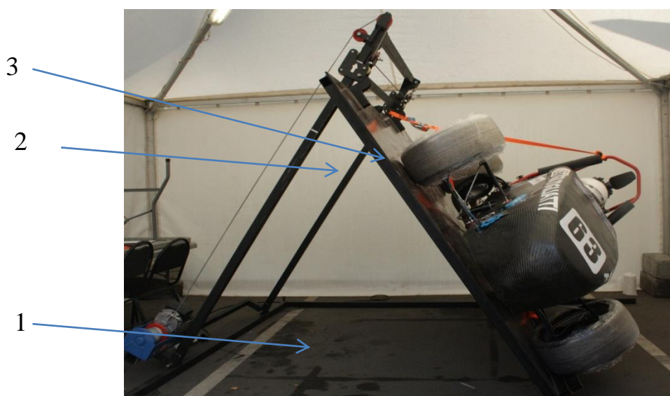
1- каркас рамы; 2 – каркас платформы; 3 – ограничитель
