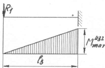
Рисунок 3.8 - Схема для проверочного расчета на прочность кронштейна крепления платформы
