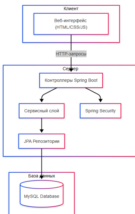
Рисунок 9 – Обобщенная архитектура системы
