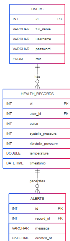
Рисунок 10 – ER-диаграмма базы данных
