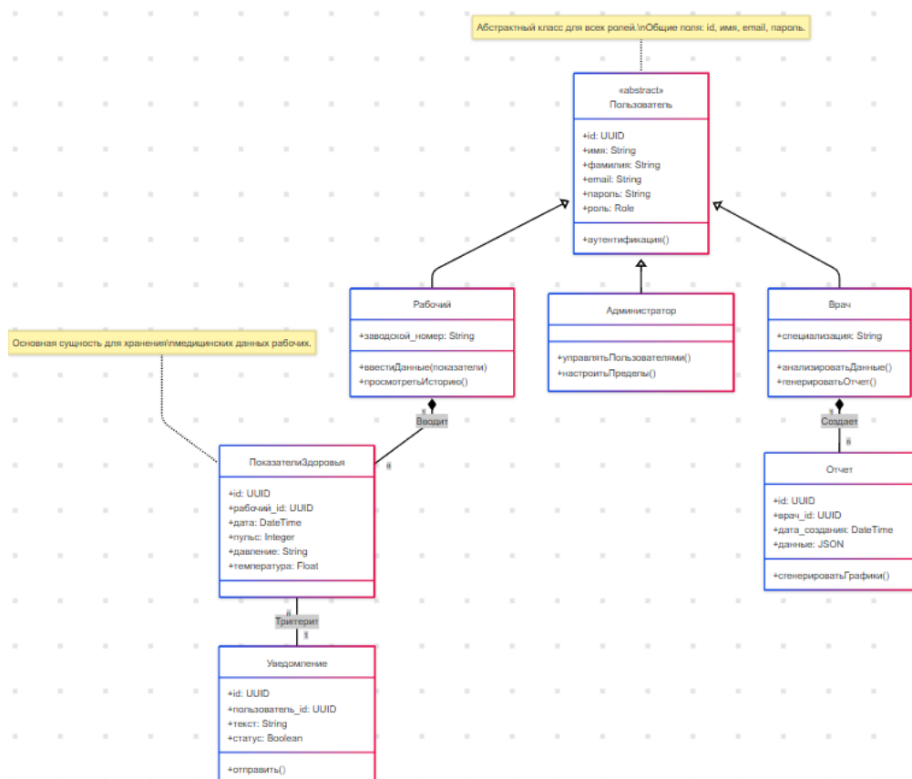
Рисунок 11 – Представление диаграммы классов
