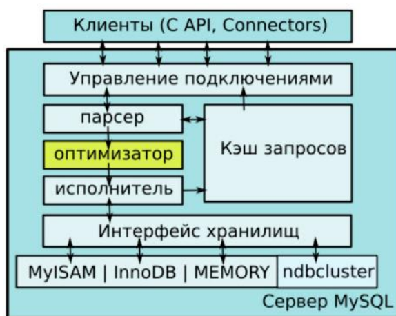
Рисунок 6 – Компоненты MySQL
