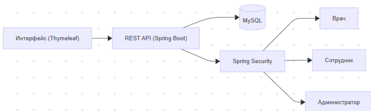
Рисунок 5 – Архитектура системы
