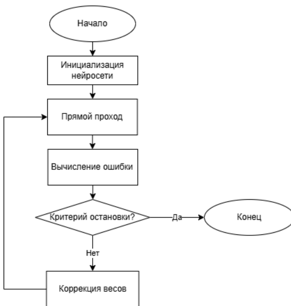
Рисунок 4 - Блок-схема нейросетевого алгоритма
