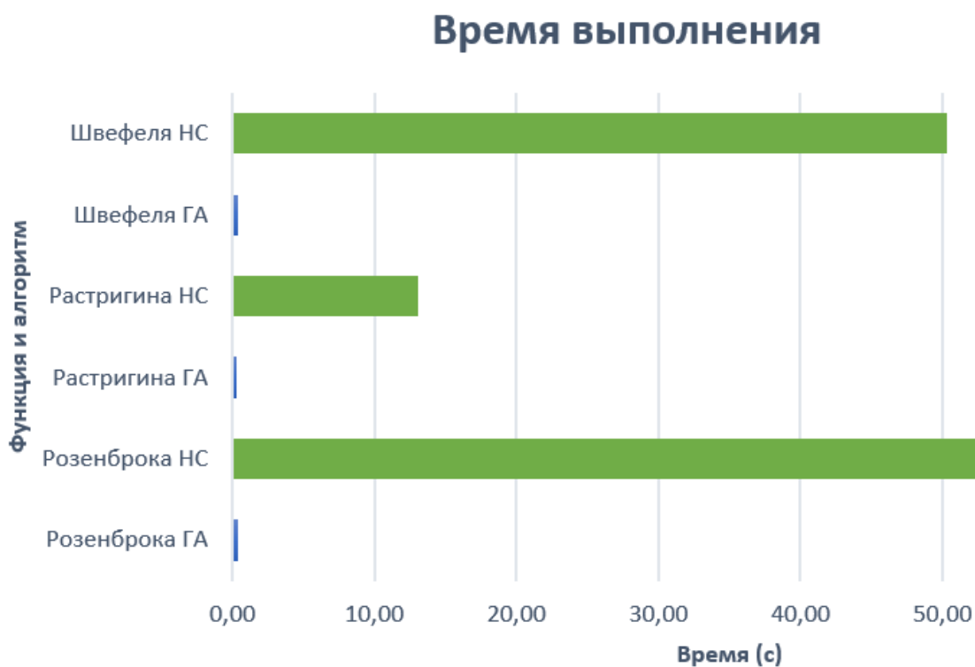
Рисунок 16 – Время выполнения тестовых функций для ГА и НС
