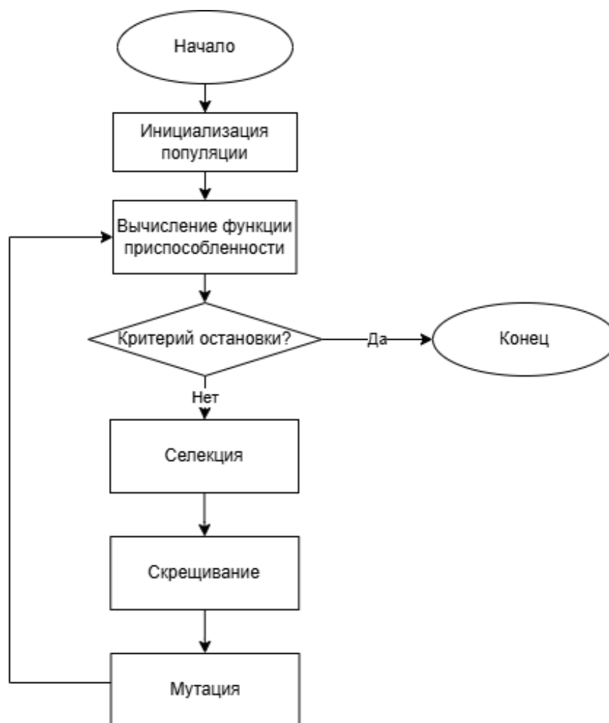
Рисунок 3 – Блок-схема генетического алгоритма
