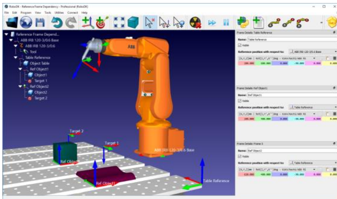
Рисунок 18 – Основное окно среды RoboDK
