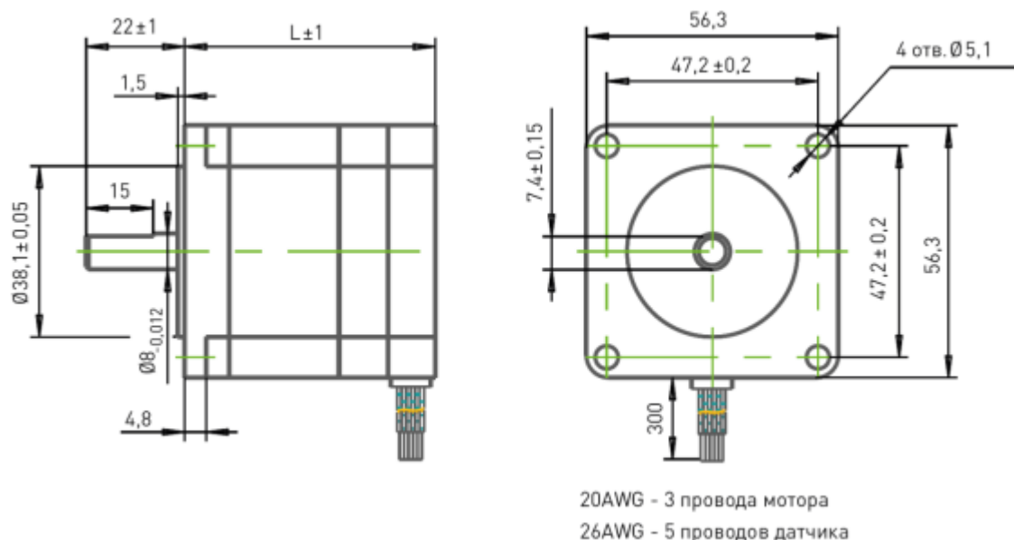
Рисунок 4 – Чертеж привода форм-фактора PL57BLF
