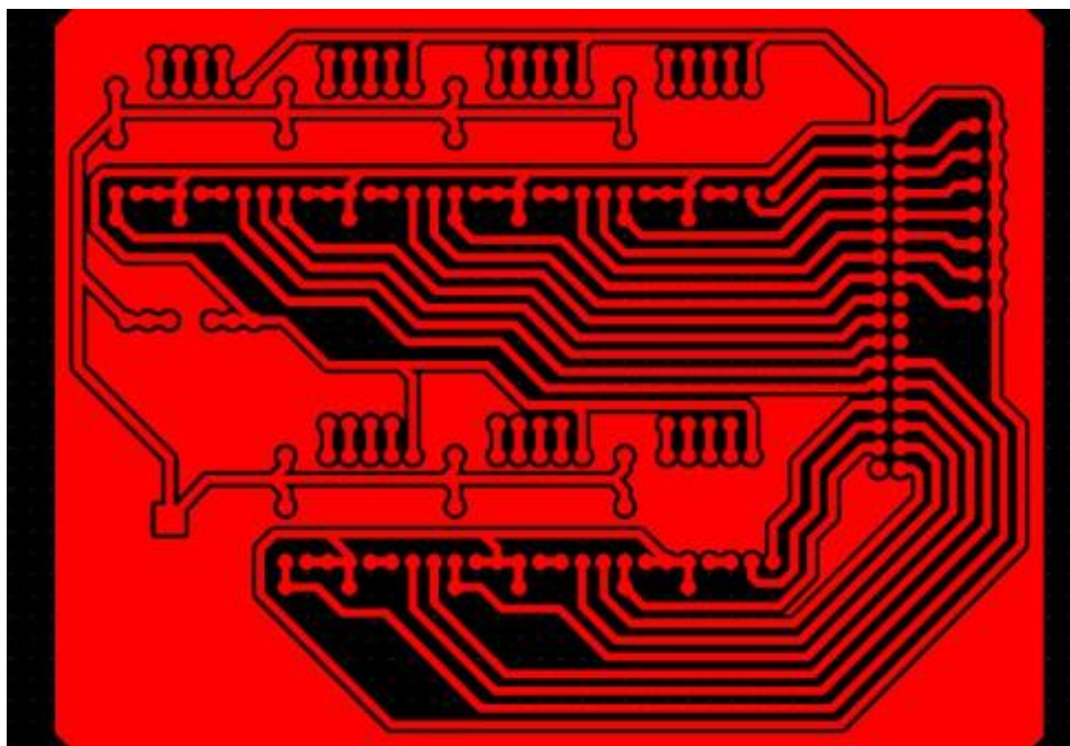
Рисунок 11 – Разведение 7 осевой Shield-платы для Arduino Mega
