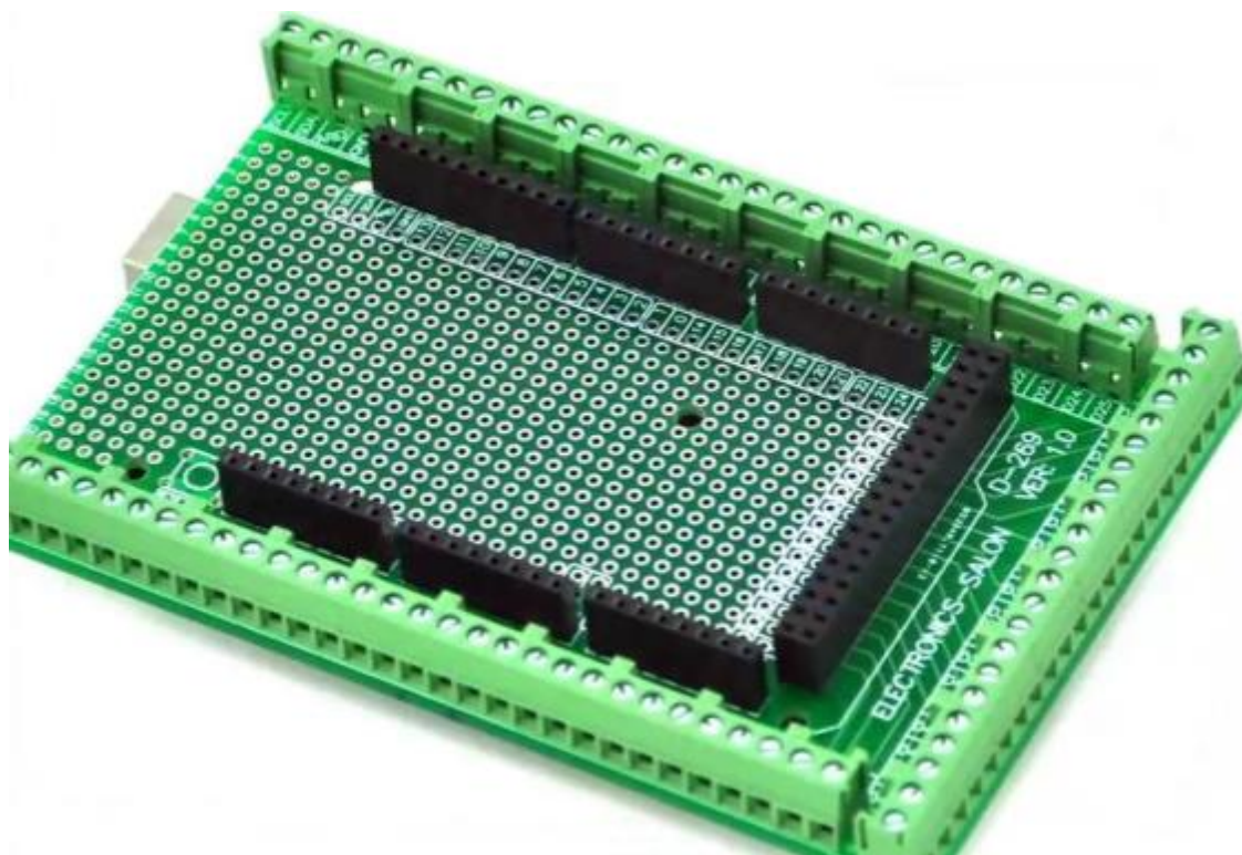
Рисунок 2 – Терминальный адаптер
