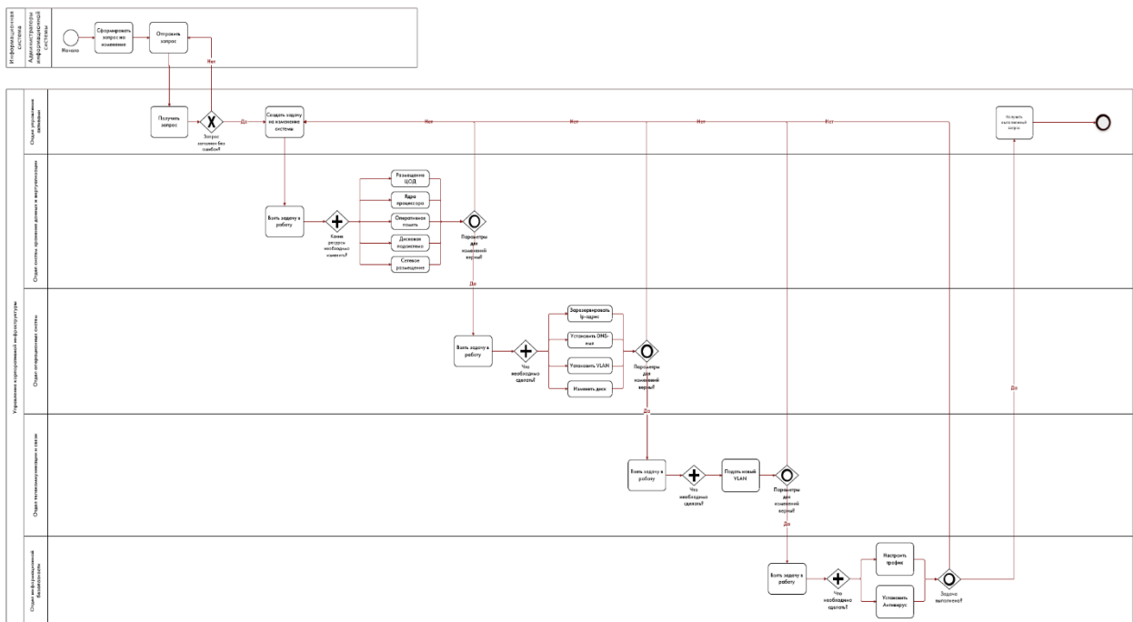
Рисунок 9 – Диаграмма дорожек процесса изменения ресурсов системы КАК ЕСТЬ
