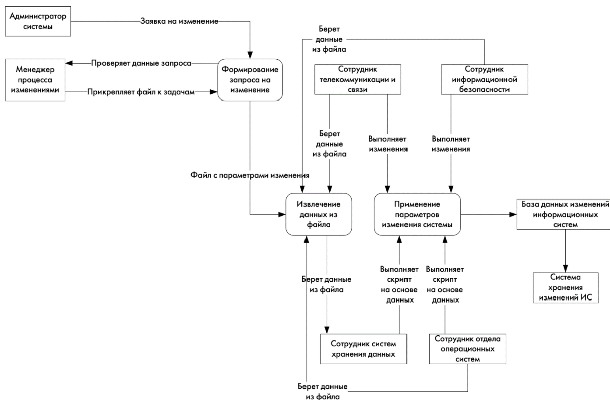
Рисунок 12 – Диаграмма потока данных, которые проходят через систему
