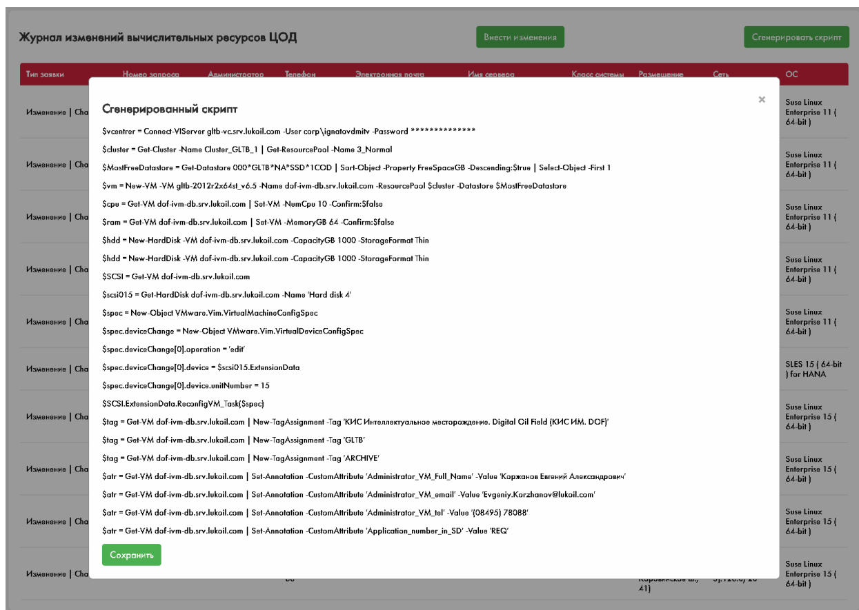
Рисунок 18 – Окно сгенерированного скрипта перед его сохранением в формате .ps1
