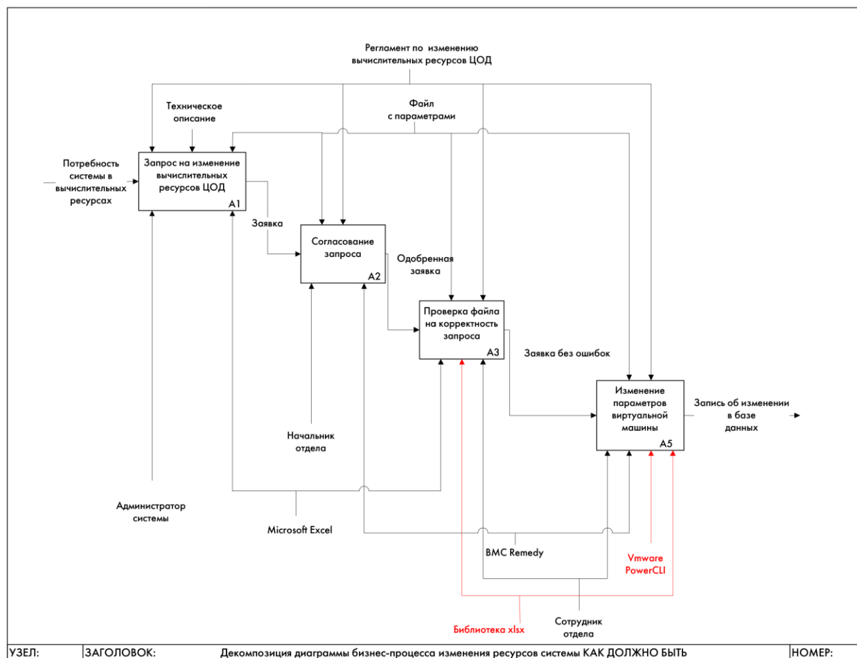
Рисунок 10 – Декомпозиция диаграммы бизнес-процесса изменения ресурсов системы КАК ДОЛЖНО БЫТЬ
