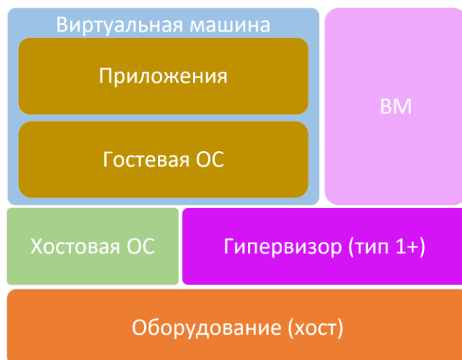
Рисунок 3 – Схема гипервизора гибридного типа
