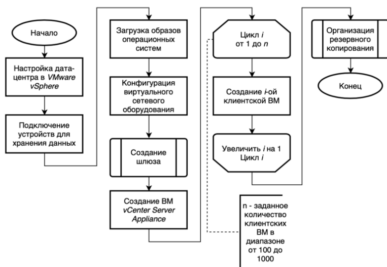
Рисунок 4 – Блок-схема метода развертывания безопасной виртуальной инфраструктуры (автор – Челнокова А.В.)
