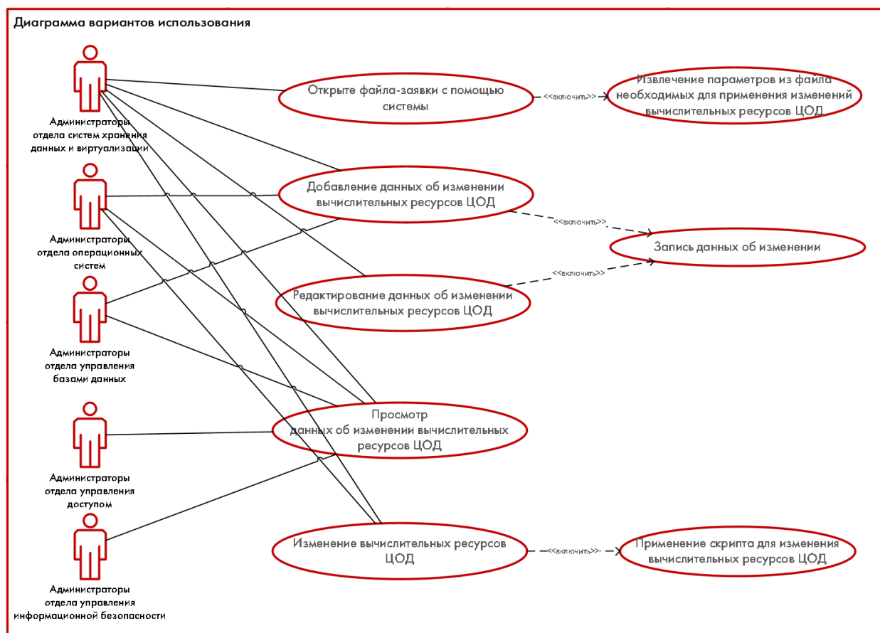
Рисунок 13 – UML-диаграмма вариантов использования
