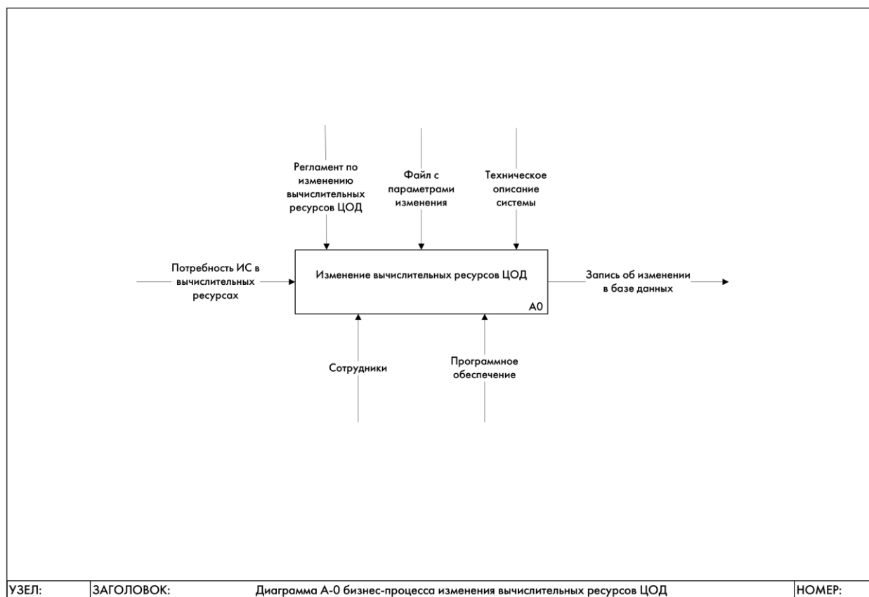
Рисунок 7 – Диаграмма А-0 бизнес-процесса изменения вычислительных ресурсов ЦОД
