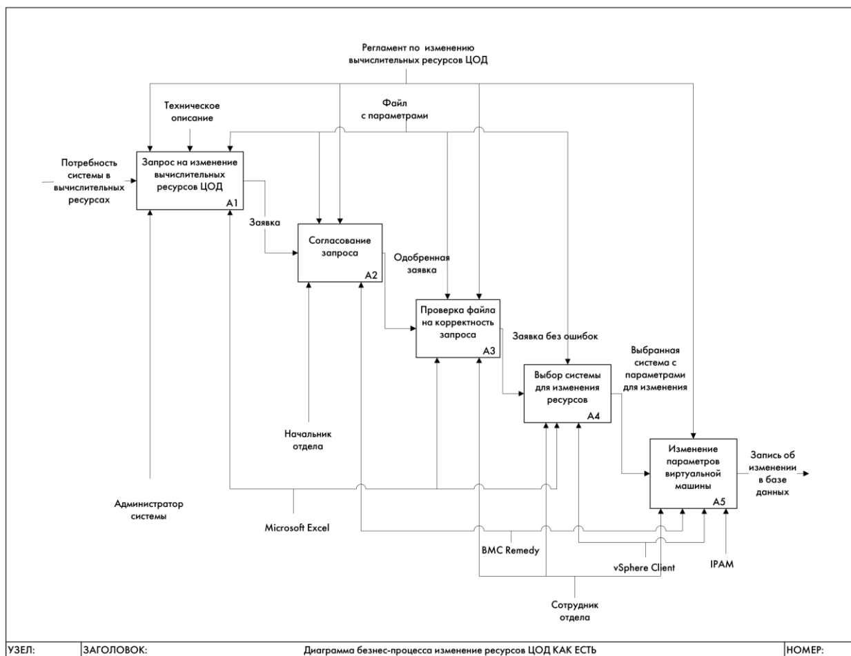
Рисунок 8 – Декомпозиция диаграммы бизнес-процесс изменения ресурсов системы КАК ЕСТЬ
