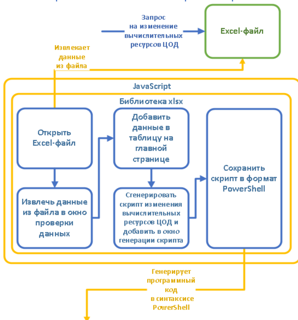
Рисунок 14 – Автоматизация процесса сбора и систематизации данных запроса с использованием алгоритма парсинга
