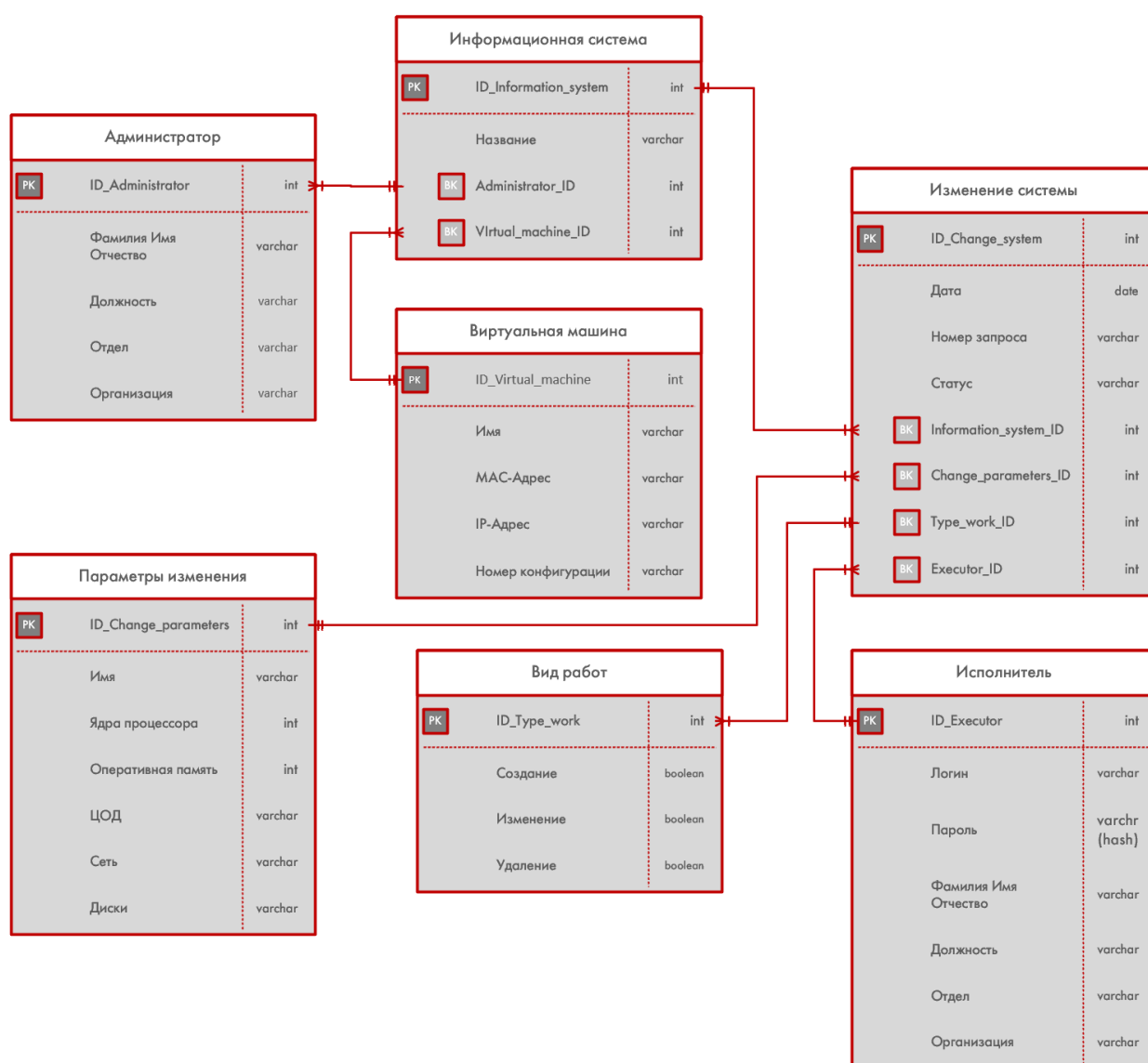
Рисунок 22 – Схема базы данных хранения информации об изменении вычислительных ресурсов ЦОД.
