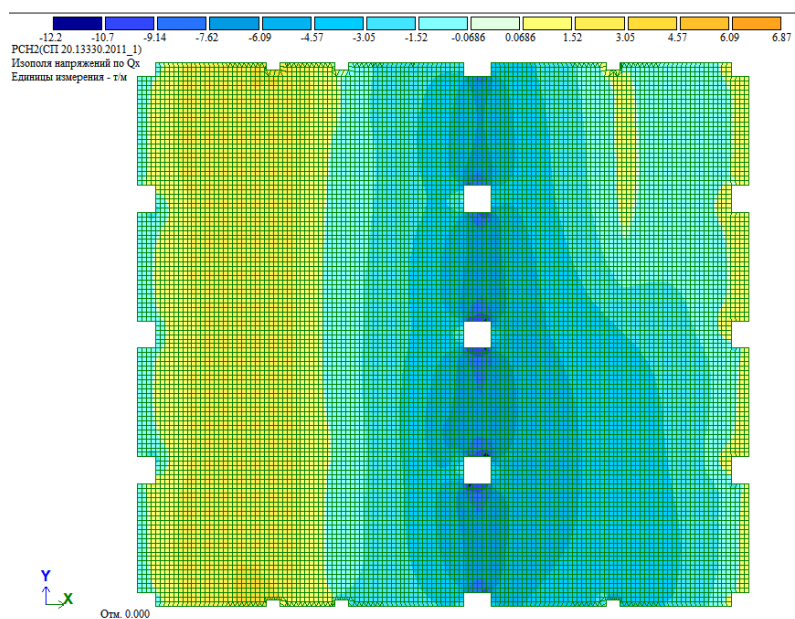
Рисунок 15 – Изополя напряжений по Q_x
