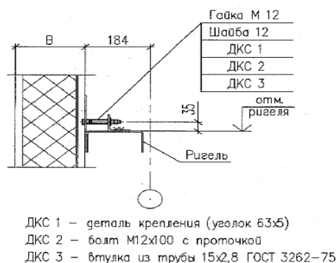
Рисунок 21 – Крепление панелей.
