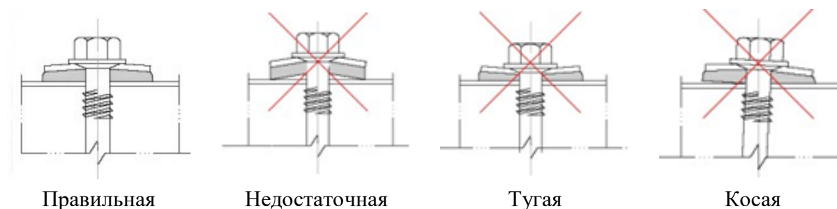
Рисунок 23 – Варианты крепление панелей винтами-саморезами
