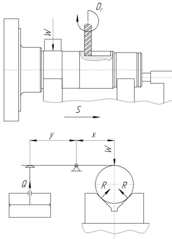
Рисунок 3 – Расчетная схема для определения усилия закрепления
