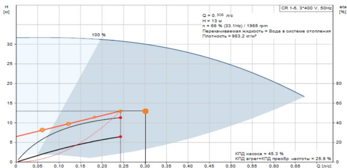
Рисунок 6 – характеристика насоса
