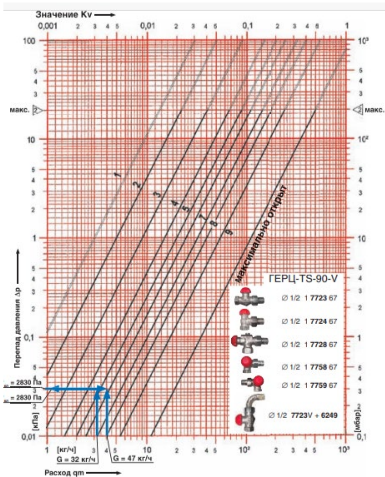
Рисунок 2 – Характеристика балансировочного клапана
