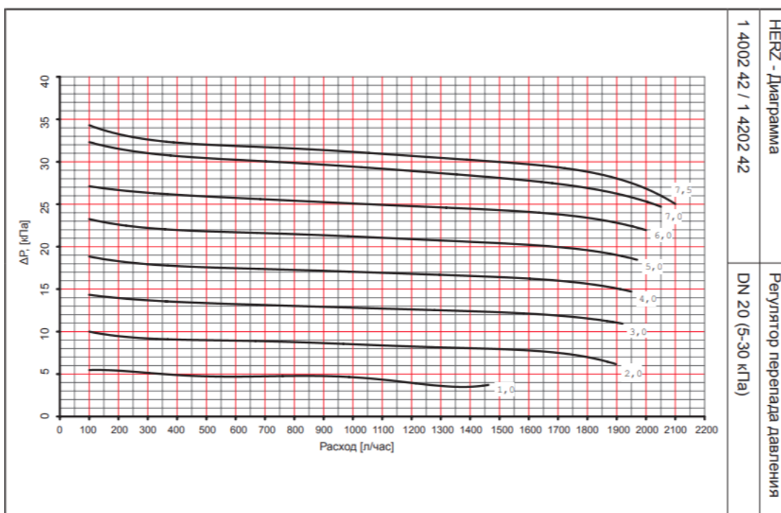
Рисунок 3 – Характеристика регулятора давления ГЕРЦ
