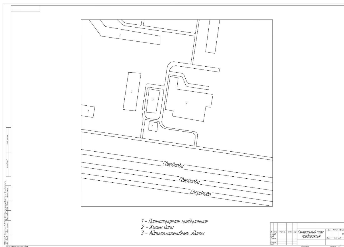
Рисунок 1 – Генеральный план предприятия
