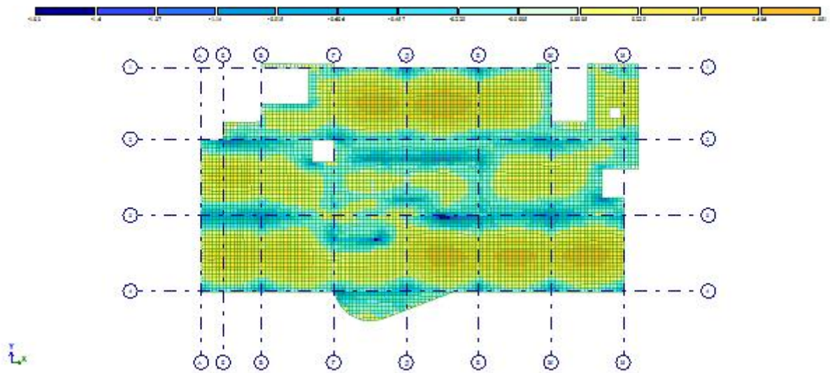
Рисунок 5- Плита перекрытия на отм. +3,720 Мозаика напряжений \mu_y
