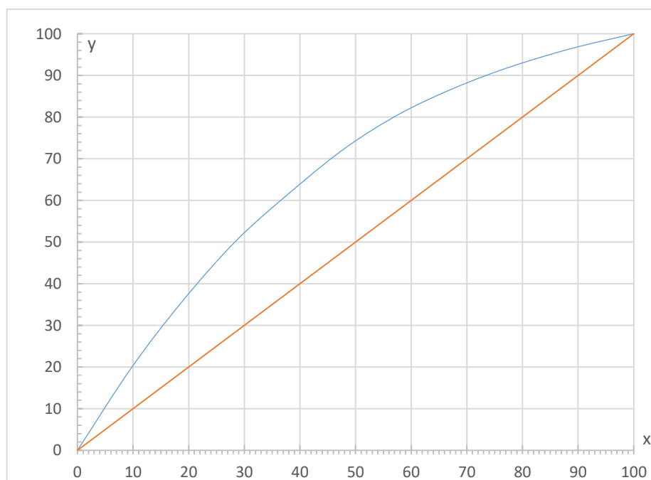
Рисунок 14 – Равновесный состав жидкости и пара
