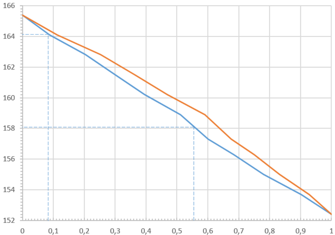
Рисунок 10 – Диаграмма t-x, y
