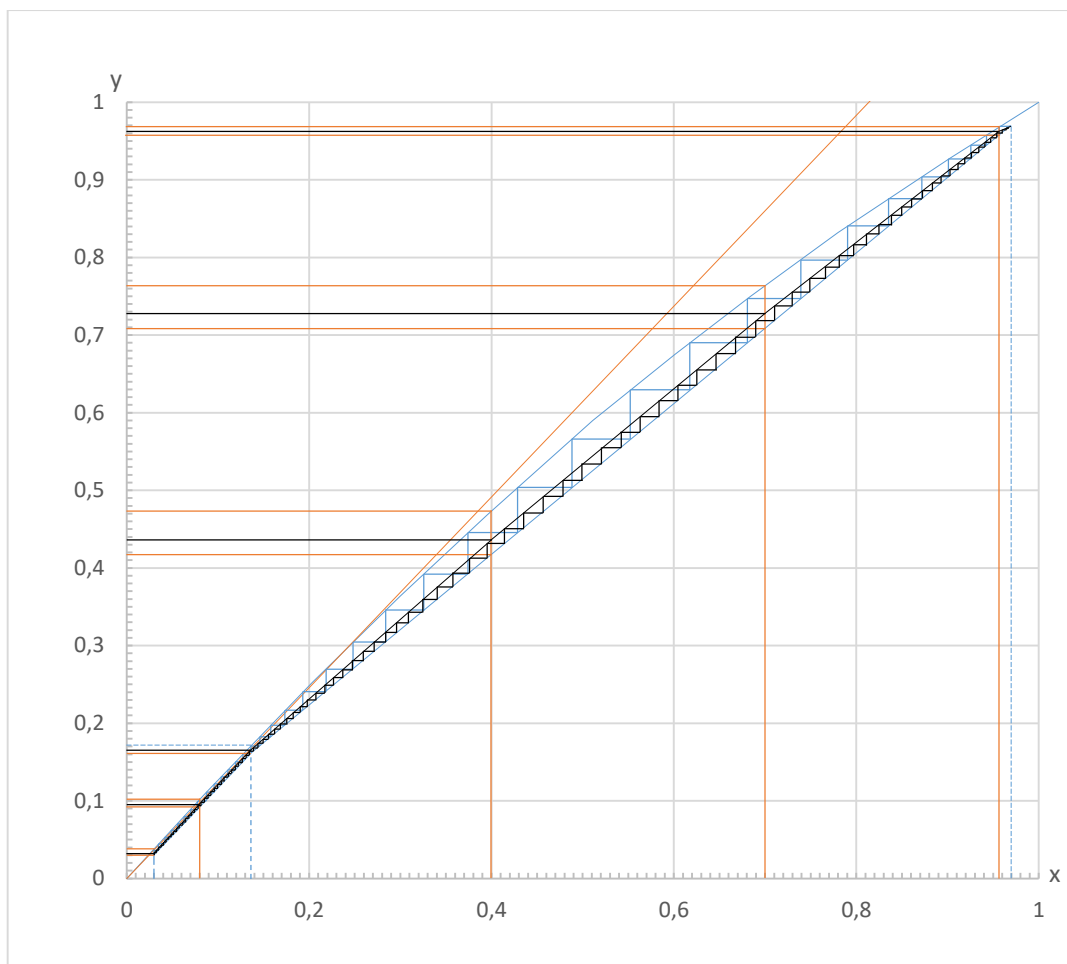
Рисунок 12 – Построение кинетической кривой и определение числа действительных тарелок
