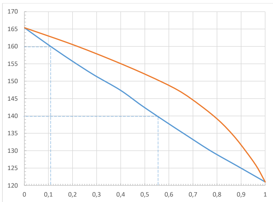
Рисунок 16 – Диаграмме t–x, y
