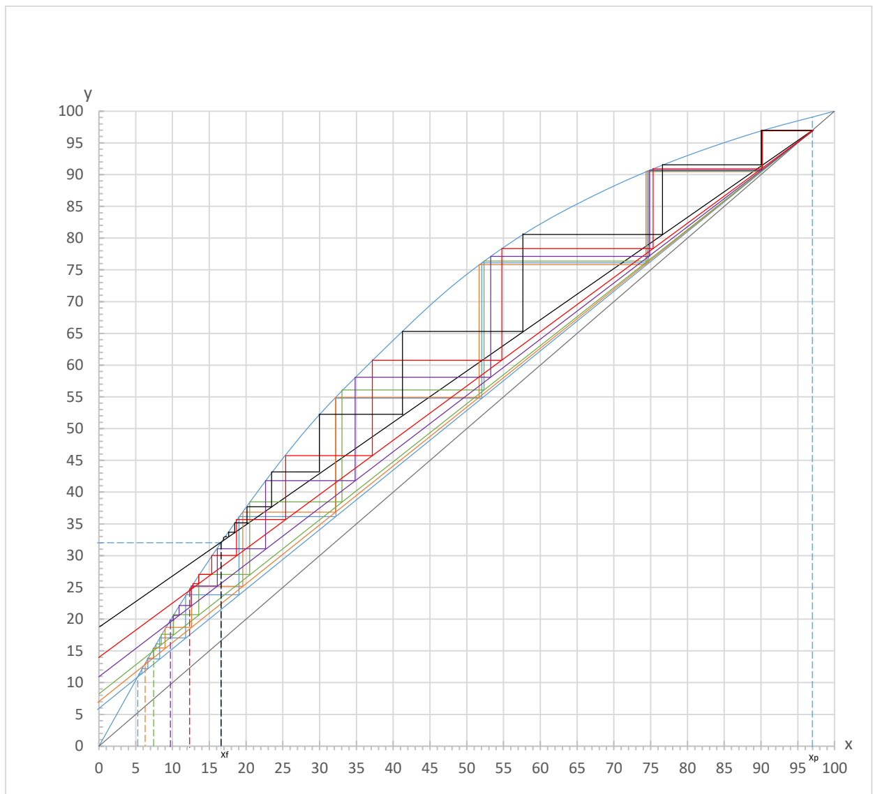
Рисунок 15 – Построение числа единиц переноса
