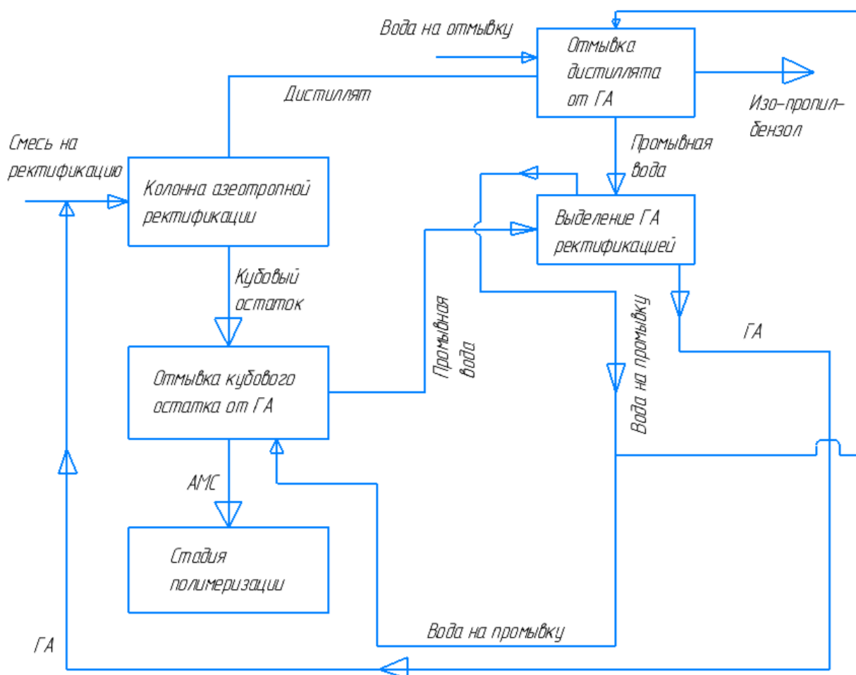
Рисунок 6 - Блок схема очистки альфа-метилстирола азеотропной ректификацией
