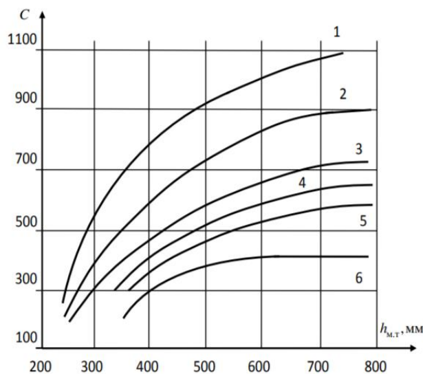
Рисунок 11 – Зависимость коэффициента C от расстояния между тарелками при расчете скорости пара в колонне:
