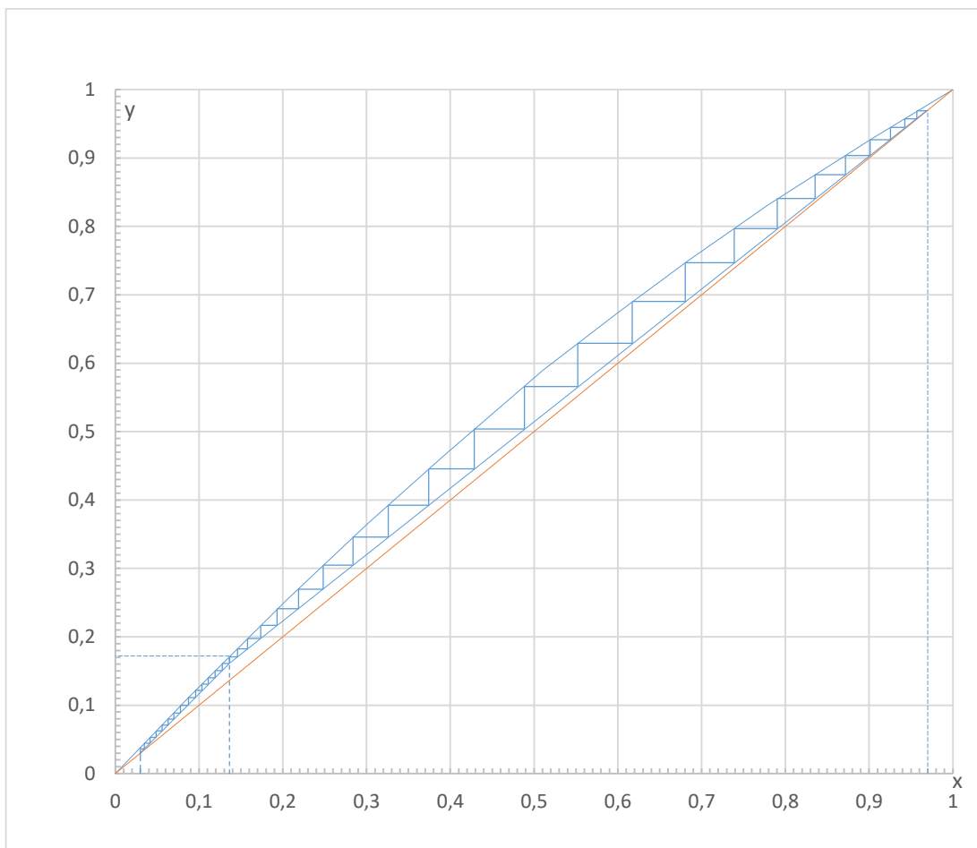
Рисунок 9 – Построение числа единиц переноса
