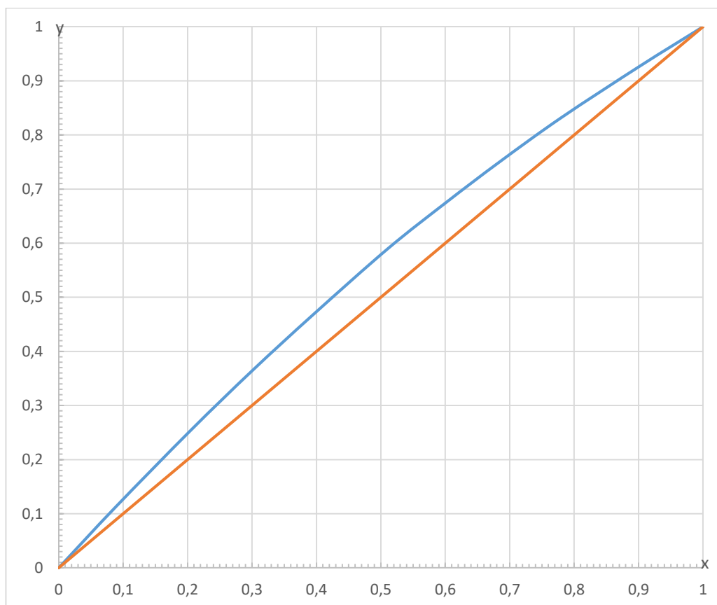
Рисунок 8 – Равновесный состав жидкости и пара
