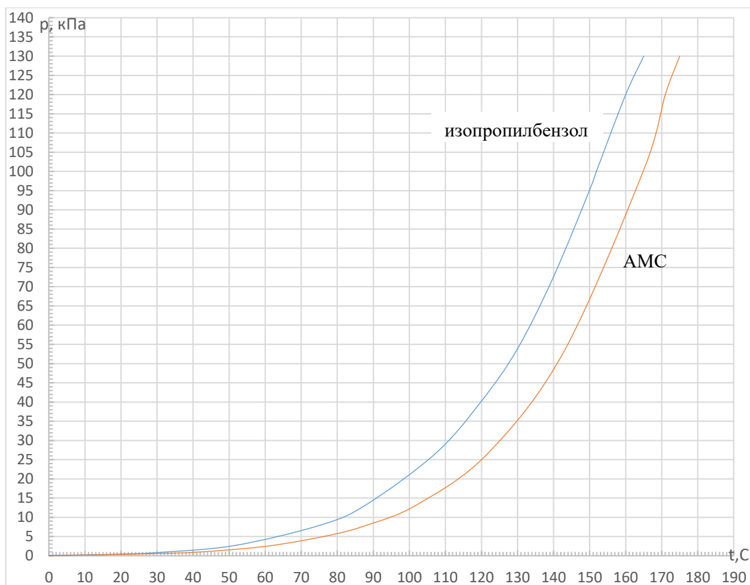
Рисунок 7 – Зависимости давление насыщенных паров изопропилбензола и АМС от температуры
