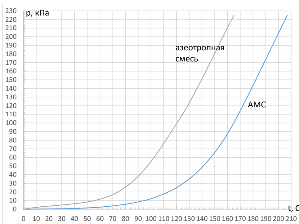
Рисунок 13 – Зависимость давления насыщенных паров компонентов от температуры
