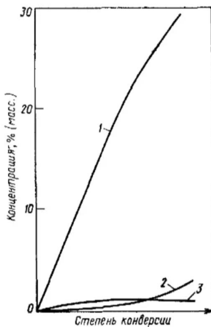
Рисунок 1 – Зависимость накопления продуктов окисления изопропилбензола от степени конверсии:
