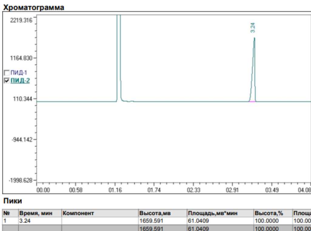
Рисунок 9 – Хроматограмма второго испытания при 60 эквивалентах
