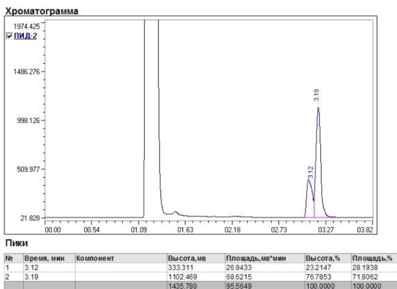
Рисунок 14 – Хроматограмма четвертого испытания при ацетонитриле
