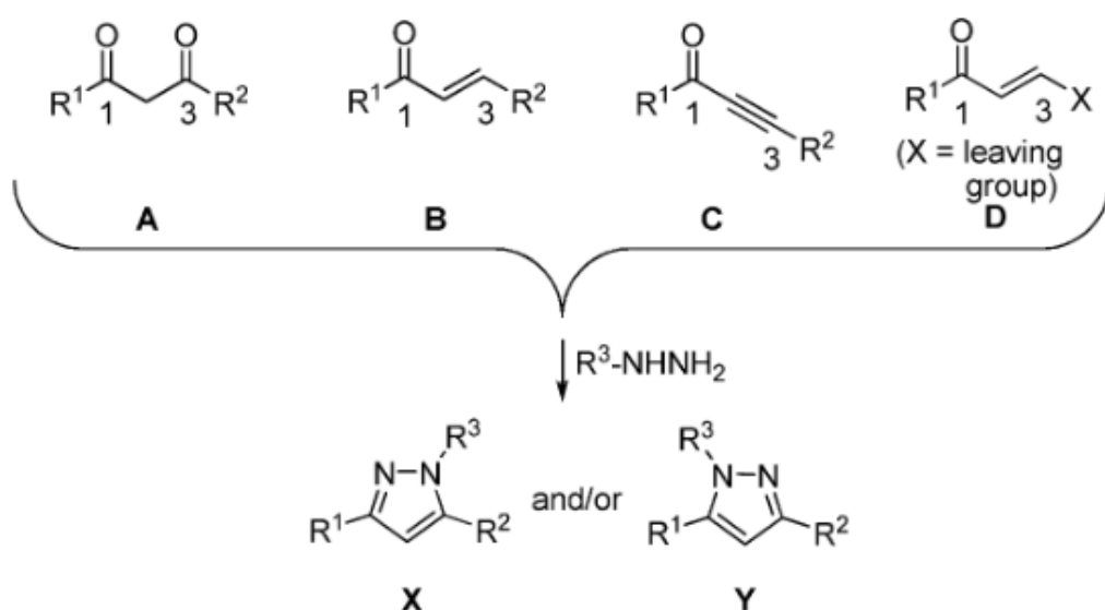
Схема 6 - Получение 3,5-дизамещенных пиразолов
