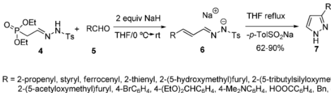
Схема 2- Синтез Сантагостина
