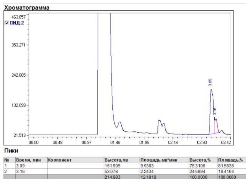
Рисунок 15 – Хроматограмма четвертого испытания при гексане
