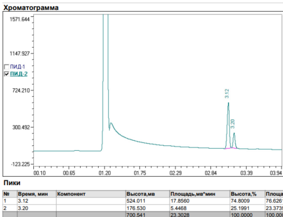
Рисунок 10 – Хроматограмма третьего испытания при 10 эквивалентах
