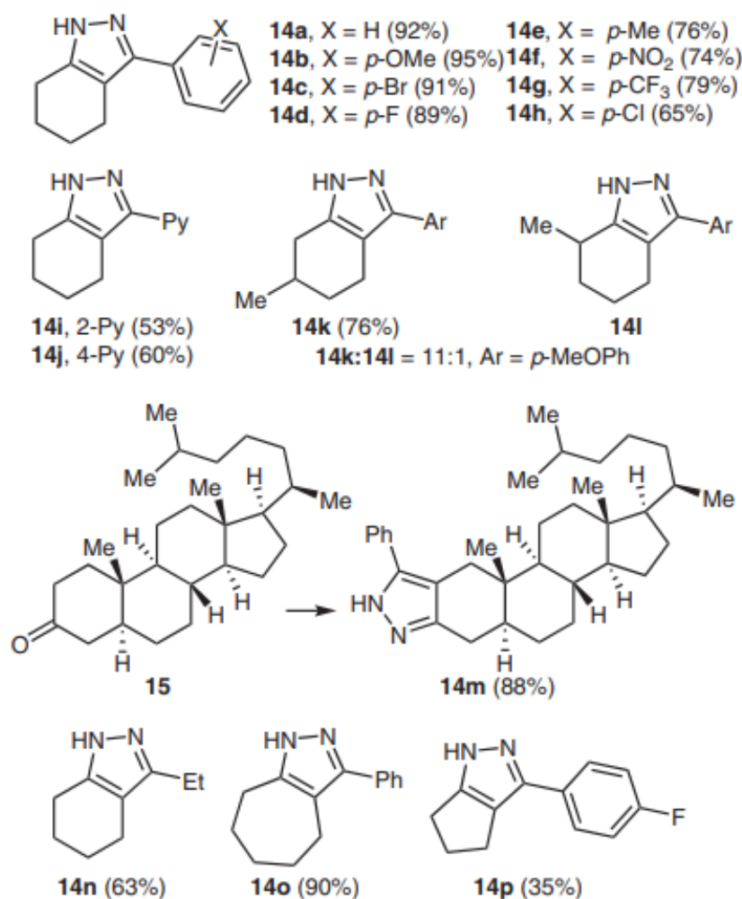
Схема 21 - Общая процедура однокомпонентного, трехкомпонентного соединения и последующего окисления бромом для синтеза пиразолов 14а–р
