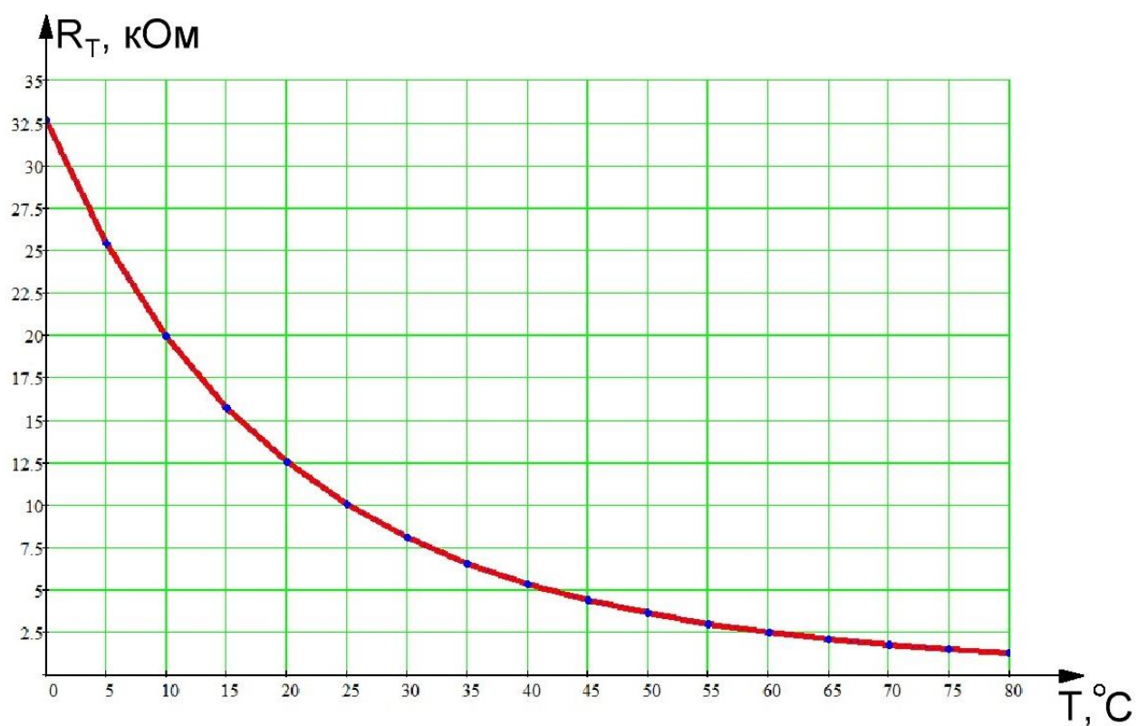
Рисунок 7 – График зависимости R_T = f(T)
