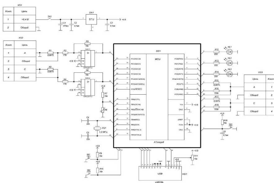
Рисунок 21 – Принципиальная электрическая схема
