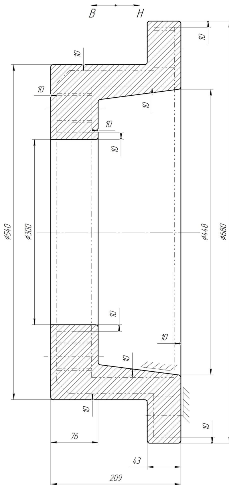
Рисунок 2 – Общий вид заготовки
