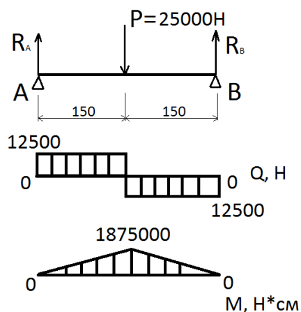
Рисунок 7 –Эпюры сил сжатияи и среза
