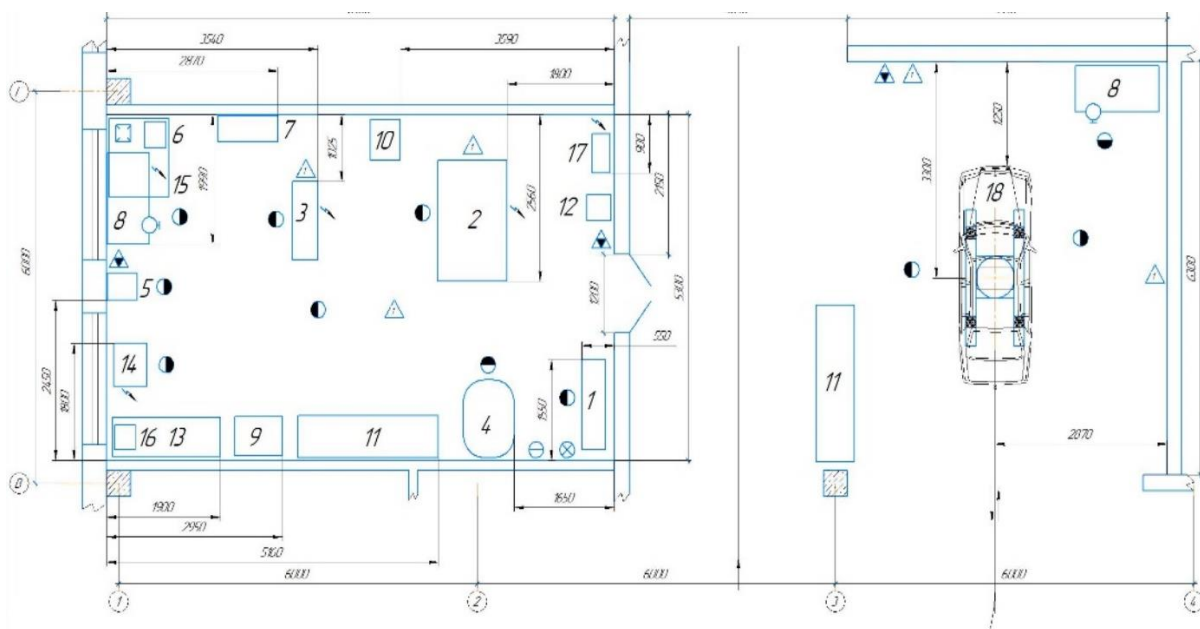
Рисунок 1 – Планировка шинного отделения
