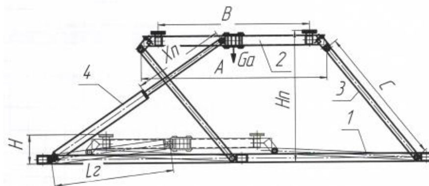
Рисунок 6 – Расчетная схема нагруженной рамы
