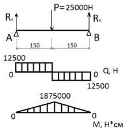
Рисунок 7 –Эпюры сил сжатияи и среза в подвижной раме
