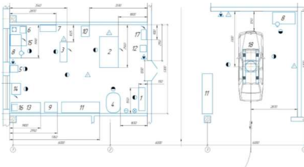
Рисунок 1 – Планировка шинного отделения
