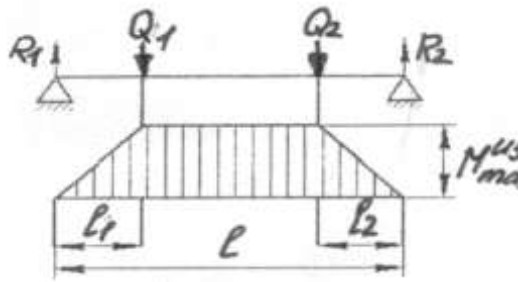
Рисунок 6 – Упрощенная расчетная схема нагруженной рамы
