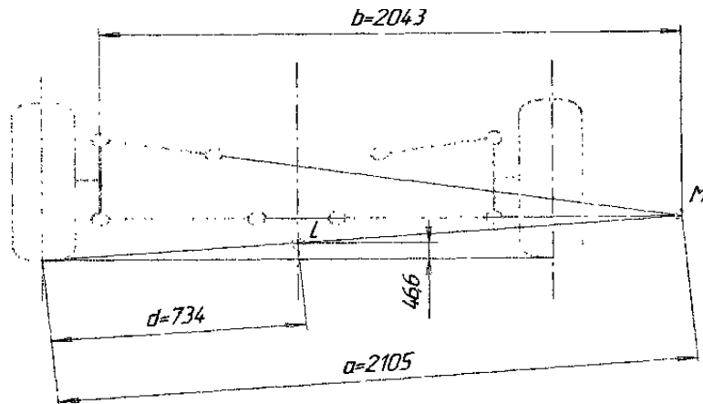
Рисунок 7 - Схема нахождения центра крена подвески
