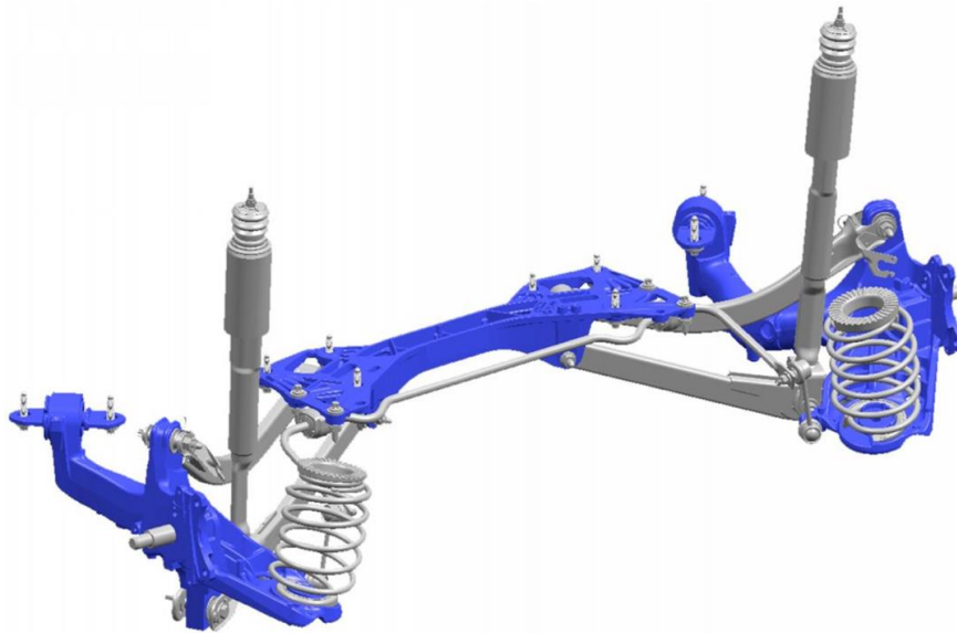
Рисунок 3 – Задняя независимая подвеска с продольными рычагами
