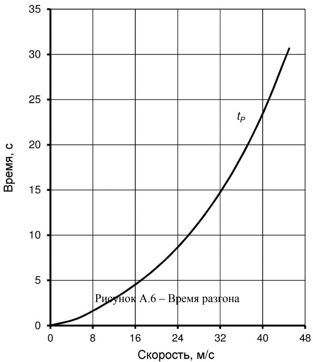
Рисунок А.6 – Время разгона
