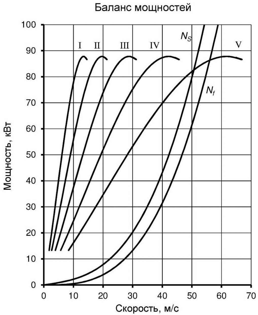
Рисунок А.2 – Баланс мощностей
