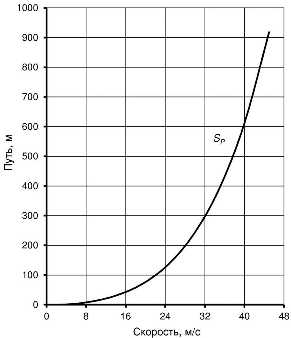
Рисунок А.7 – Путь разгона
