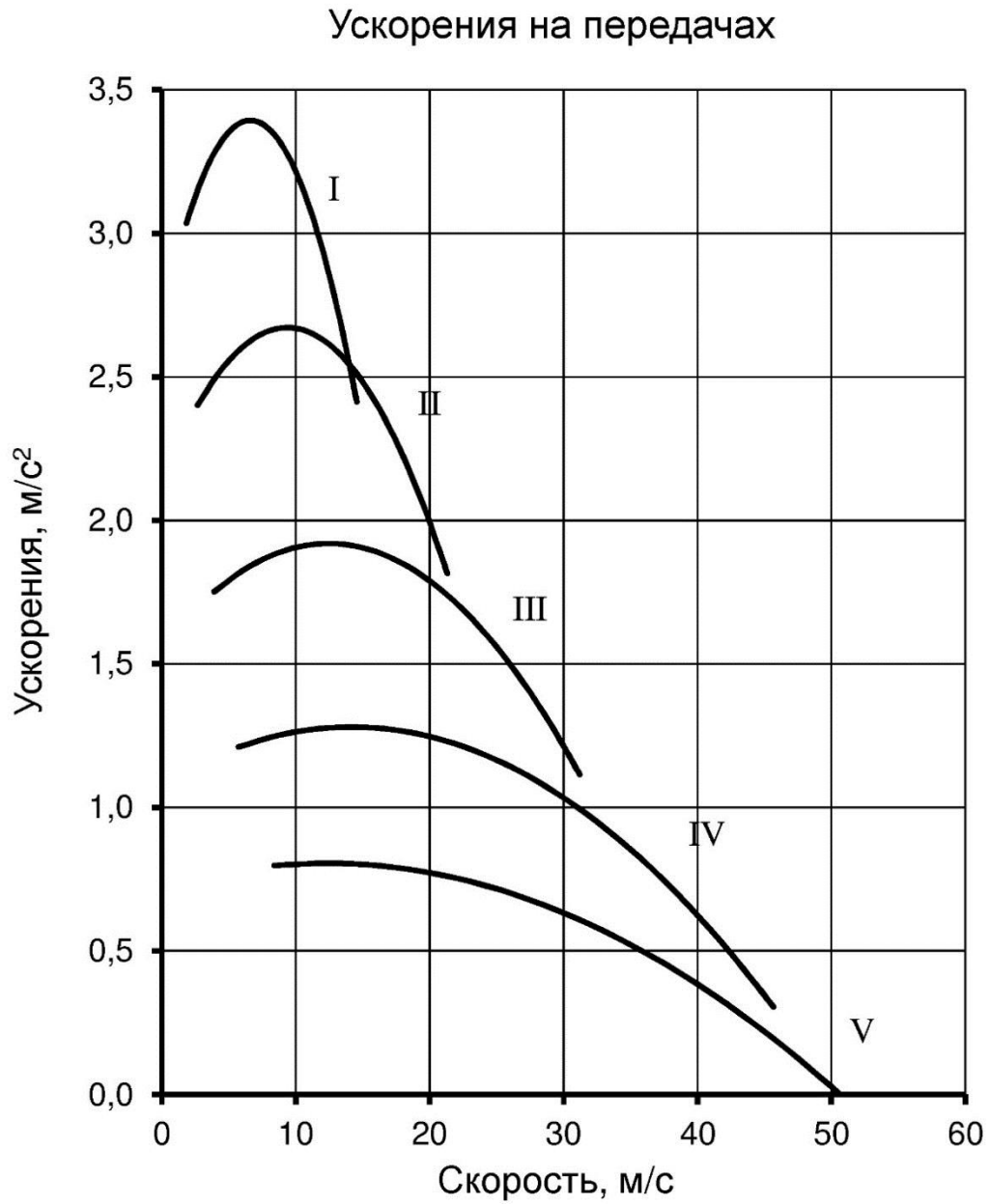
Рисунок А.5 – Ускорения на передачах
