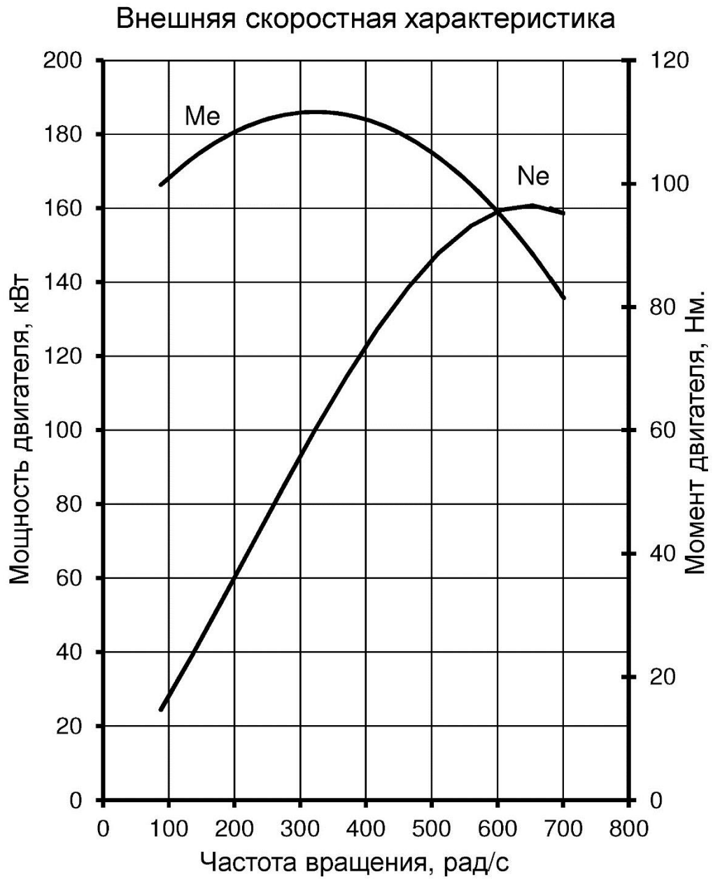
Рисунок А.1 – Внешняя скоростная характеристика
