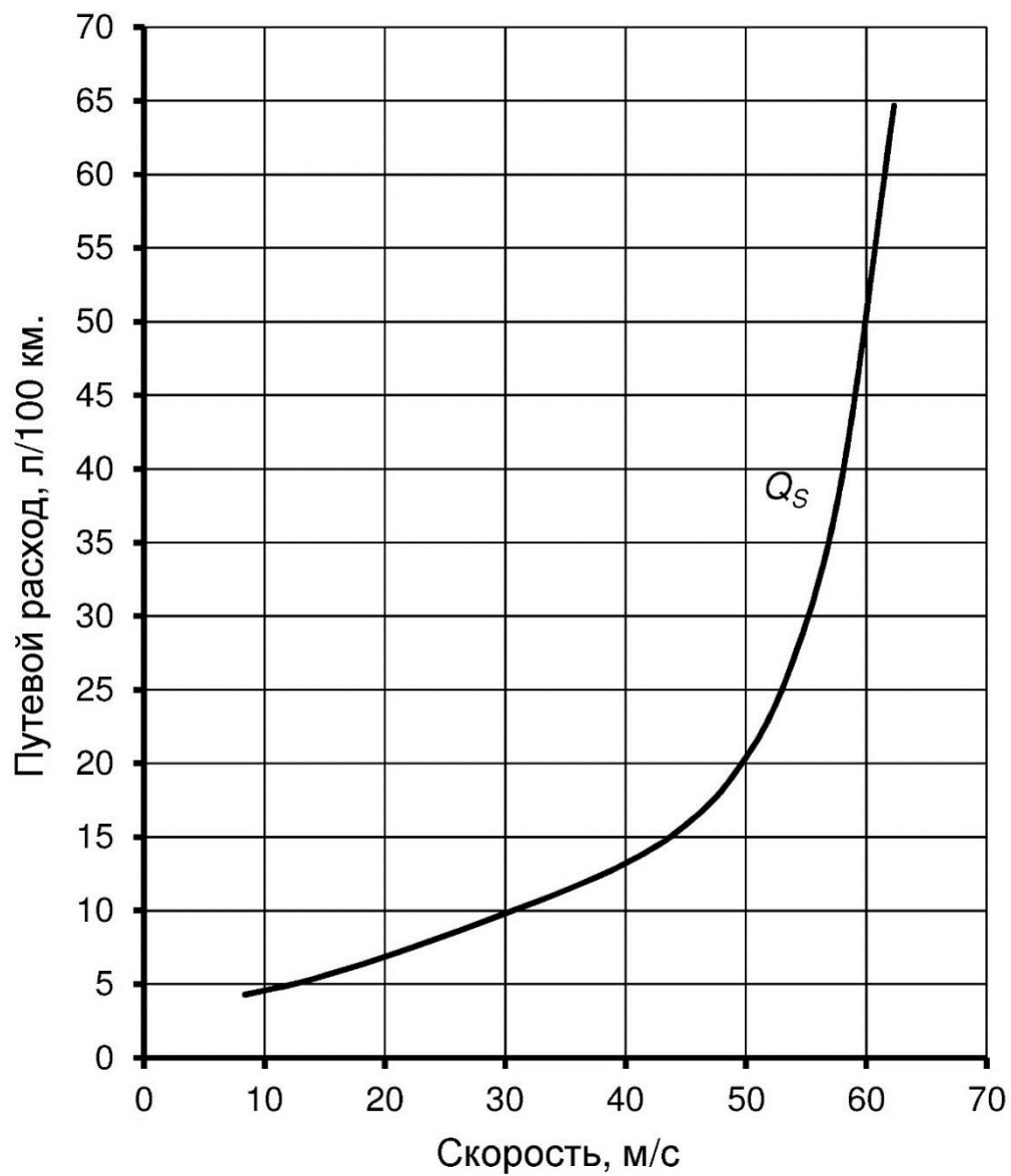
Рисунок А.8 – Путевой расход топлива
