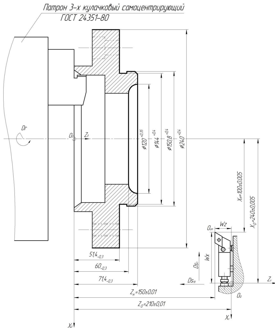
Рисунок 3 – Операционный эскиз операции 020
