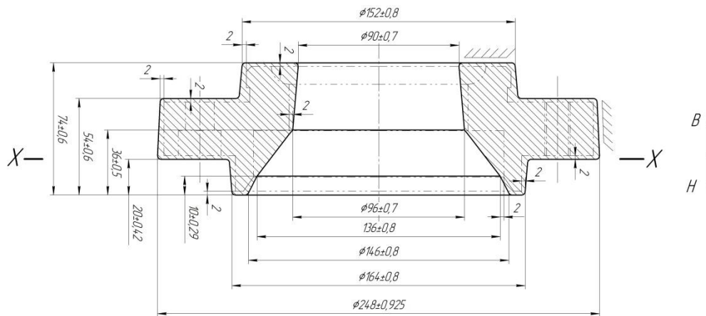
Рисунок 2 – Общий вид отливки
