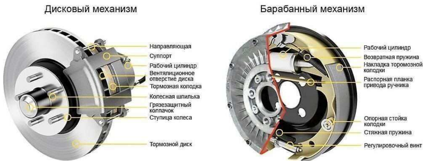
Рисунок 3 – Дисковый и барабанный тормозные механизмы
