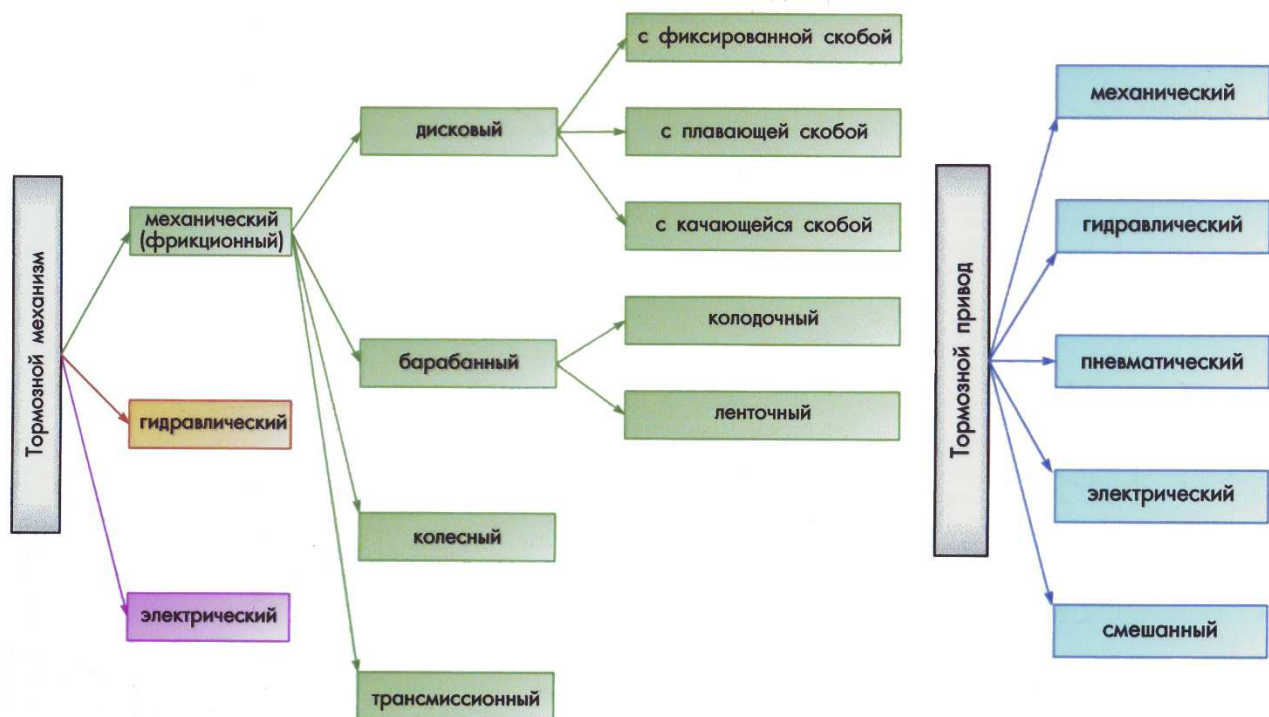
Рисунок 1 – Схема классификации тормозных механизмов и приводов
