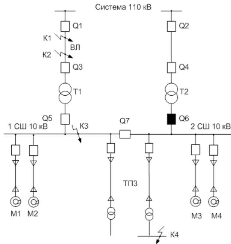
Рисунок 7 – Расчетная электросхема системы электроснабжения предприятия по выпуску металлической продукции для определения токов КЗ
