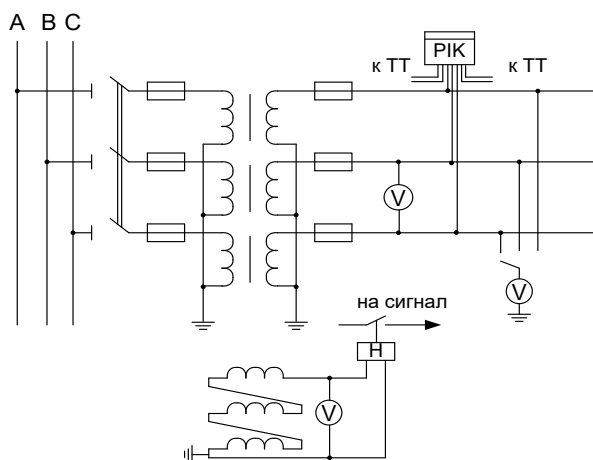
Рисунок 11 – Схема подключения ТН и КИП
