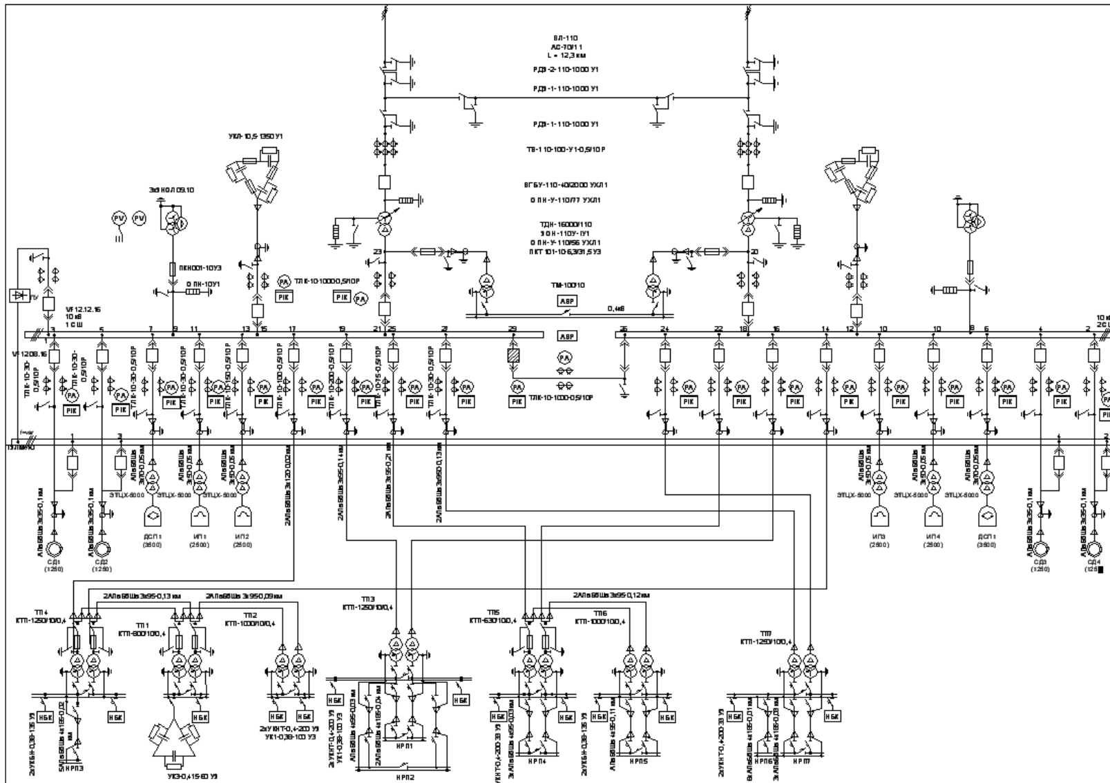
Рисунок 6 – Схема электрическая принципиальная промышленного предприятия
