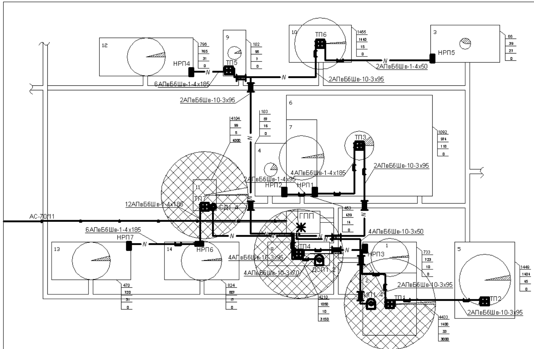
Рисунок 5 – Схема прокладки кабельных линий по территории предприятия
