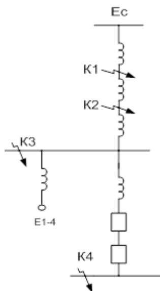
Рисунок 8 – Схема замещения
