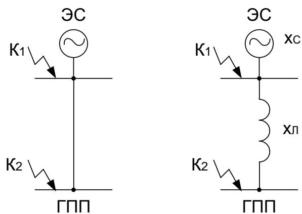
Рисунок 2 – Расчетная схема питания предприятия по выпуску металлической продукции и схема замещения
