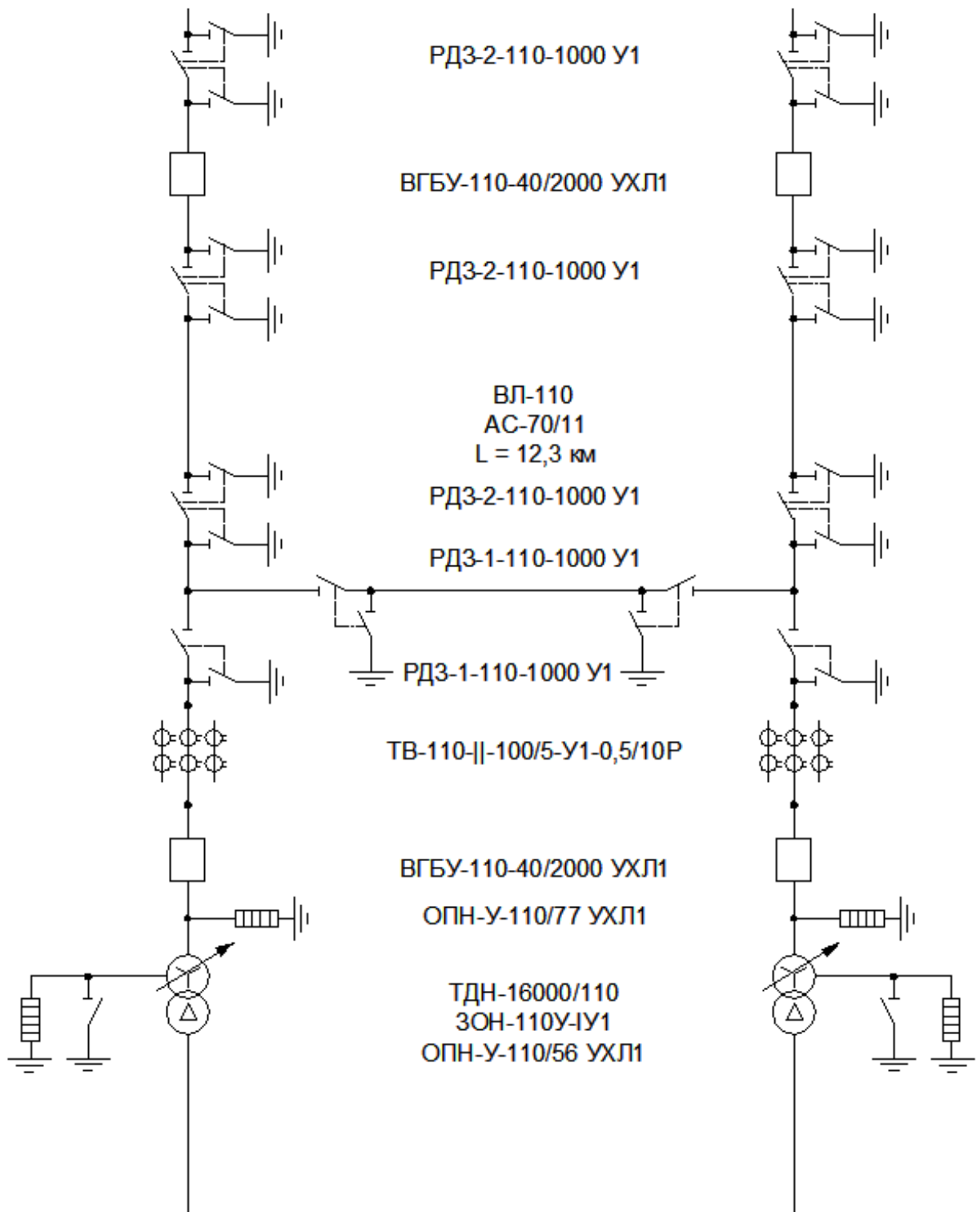
Рисунок 4 – Схема сети 110 кВ
