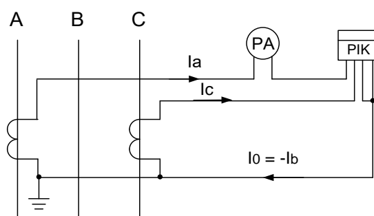
Рисунок 10 – Схема подключения ТТ и КИП
