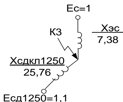
Рисунок 9 – Упрощенная схема замещения для определения ТКЗ в точке K_3
