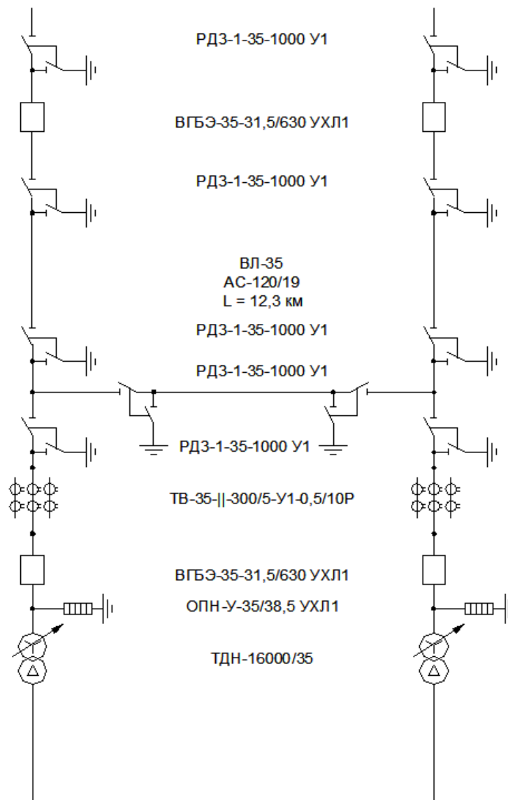
Рисунок 3 – Схема сети 35 кВ
