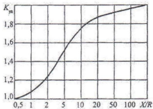
Рисунок 2 – Кривая для определения значения ударного коэффициента в зависимости от величины отношения X/R
