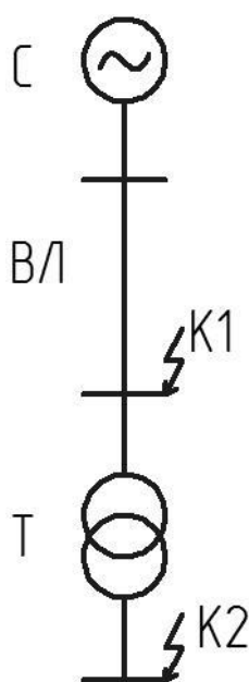
Рисунок 4 – Расчетная схема для определения значений токов КЗ на ПС «Бердянка»
