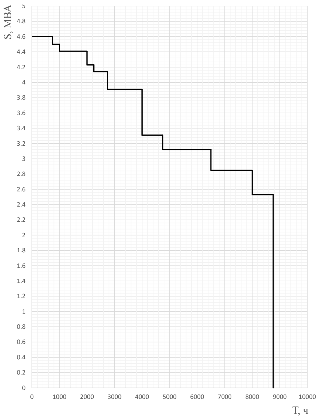
Рисунок 2 – Упорядоченный годовой график нагрузки ПС «Бердянка»
