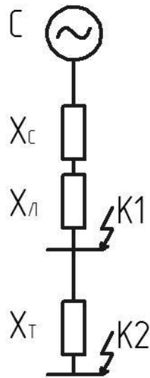
Рисунок 5 – Схема замещения для определения значений токов КЗ на ПС «Бердянка»
