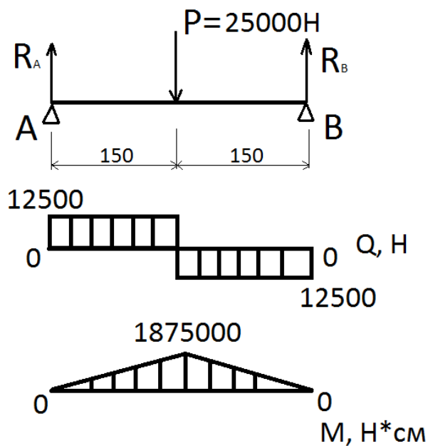
Рисунок 2.6 – Эпюры внутренних силовых факторов
