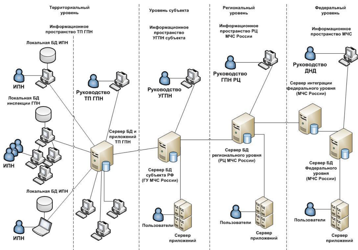
Рисунок 1 – Вариант логической схемы взаимодействия компонентов СПО ИАП
