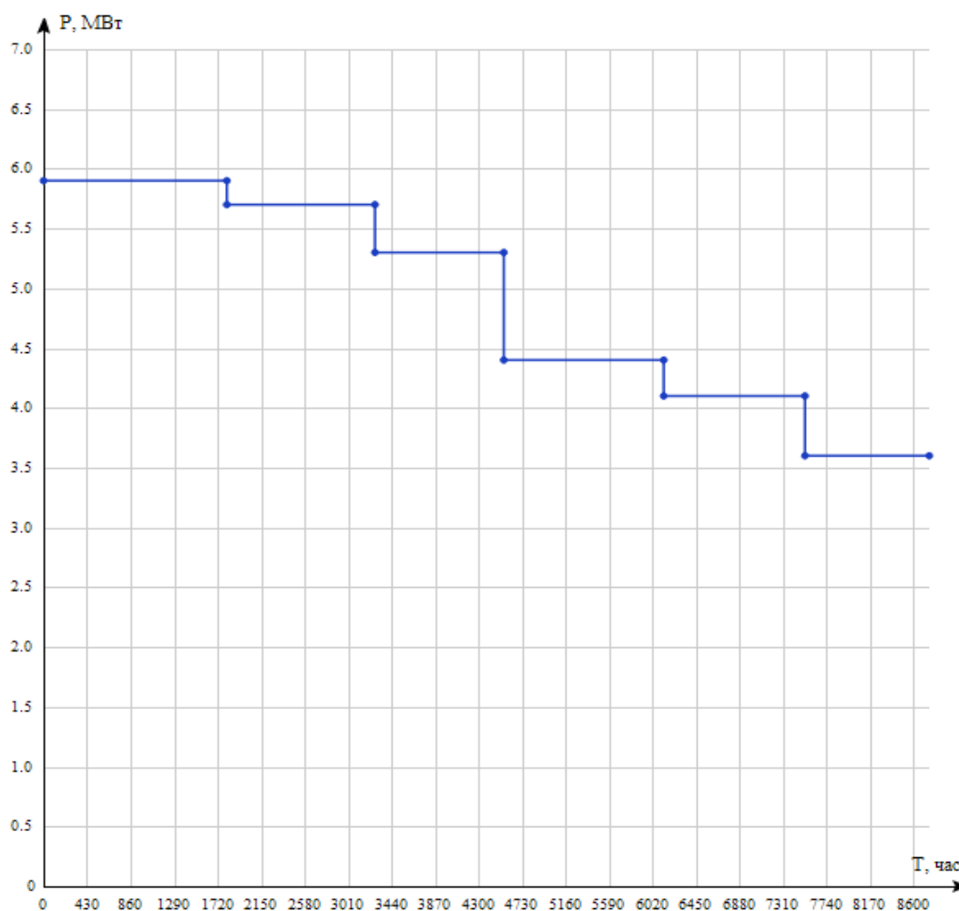
Рисунок 3 – Итоговый упорядоченный график ПС «Шушары»
