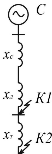
Рисунок 5 – Схема замещения для определения значений токов КЗ на подстанции «Шушары»
