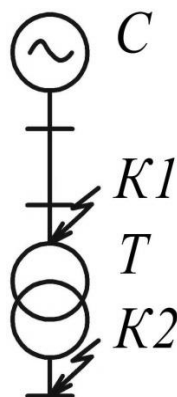
Рисунок 4 – Расчетная схема для определения значений токов КЗ на подстанции «Шушары»
