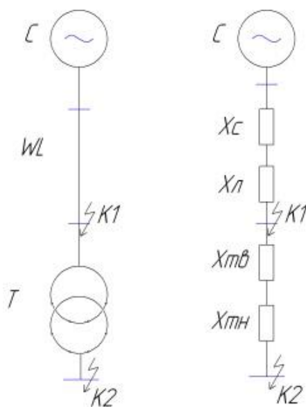
Рисунок 6.1 – Расчётная схема с основными элементами сети и ее схема замещения
