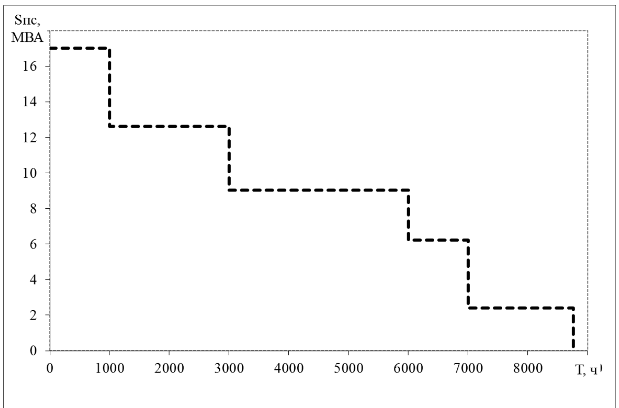
Рисунок 4.1 – Упорядоченный годовой график полной мощности главной понизительной подстанции завода
