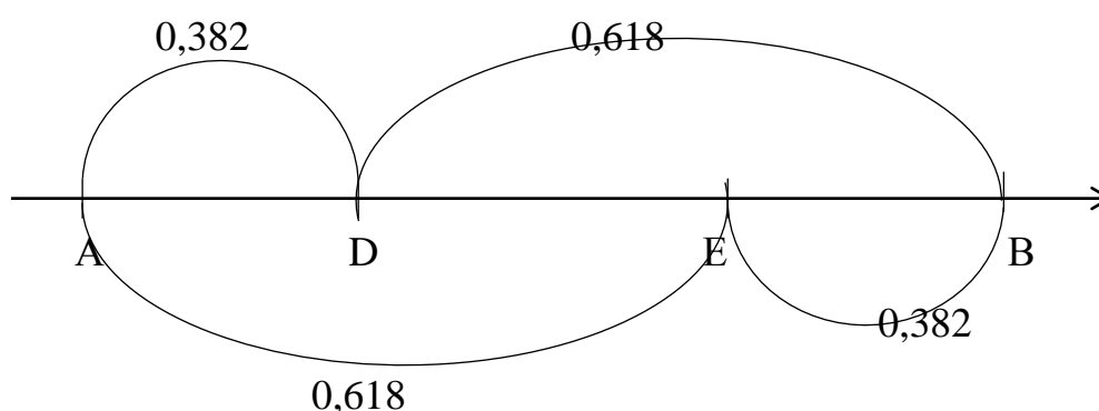
Рисунок 3.1. Геометрическая интерпретация принципа «золотого сечения»
