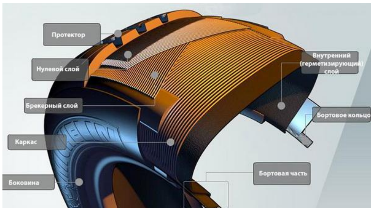
Рисунок 3.1 – Внешнее устройство автомобильной шины
