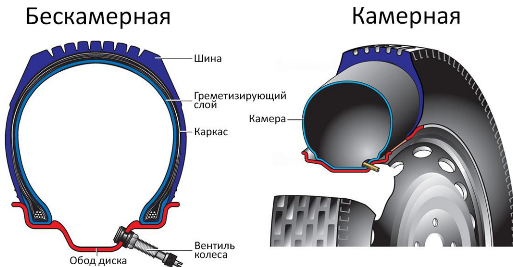
Рисунок 3.2 – Способы герметизации автомобильной шины
